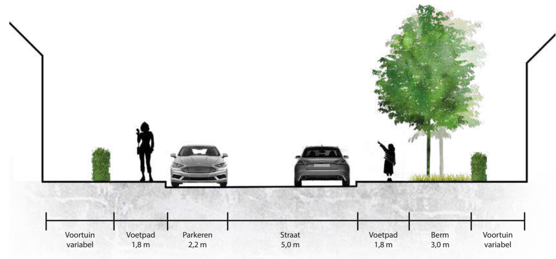
Profiel D
