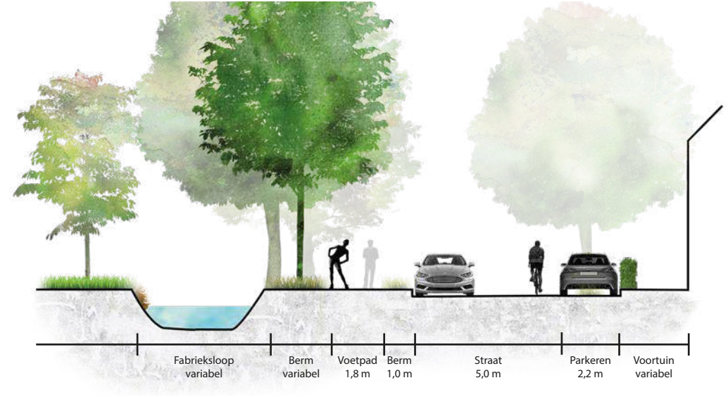
Profiel A
