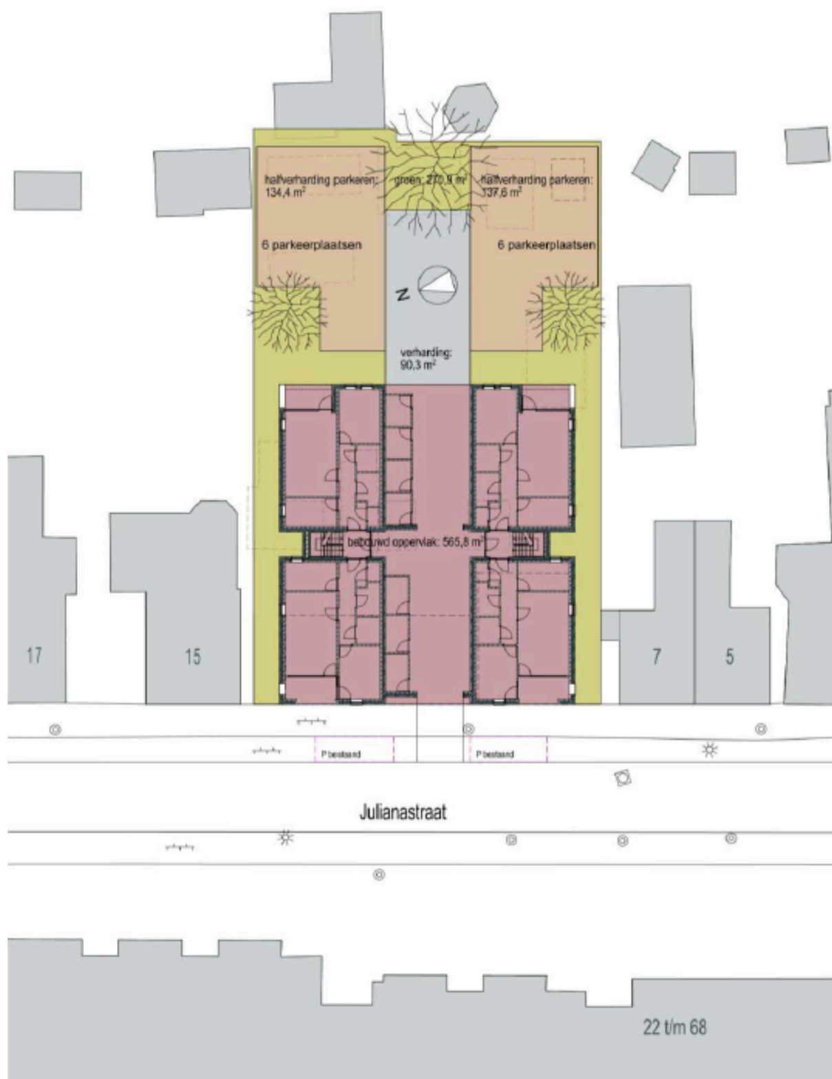
Afbeelding 6. Stedenbouwkundige planschets
