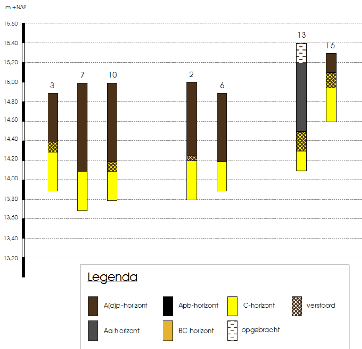
Figuur 33: Boorprofielen
