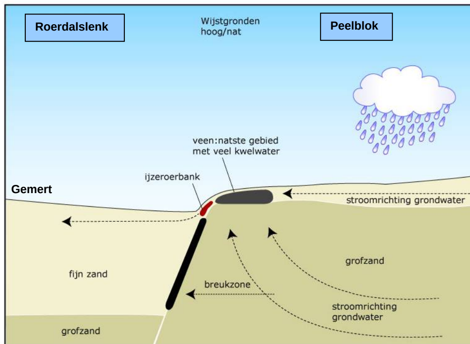
Figuur 6: Ontstaan van natte wijstgronden op een breukrand.
