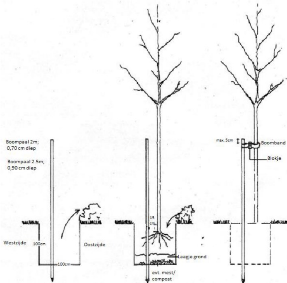
Afbeelding 7: Plantinstructie bomen
