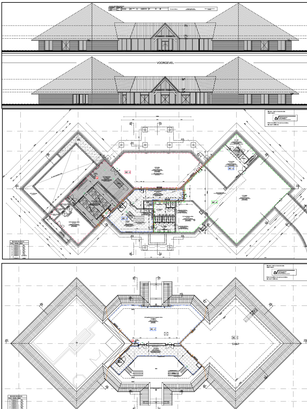
Gevelaanzichten en souterrain bestaande bezoekerscentrum natuurpoort.
