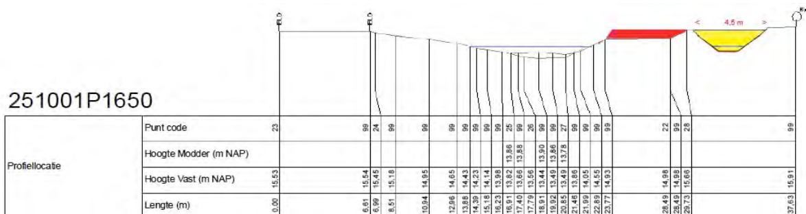
Figuur 4.24. Nieuwe doorsnede van de Peelse Loop bovenstrooms in traject I. De nieuwe bedding (geel) ligt rechts van de oude bedding, die als langgerekte vijver blijft bestaan. Lokaal wordt een deel van de oude bedding aangevuld (rood) om ruimte te scheppen voor het nieuwe versmalde profiel.
