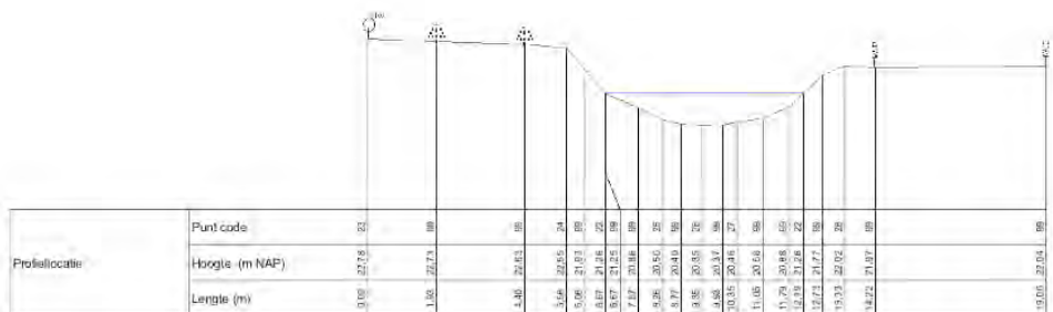
figuur 3.16. Dwarsprofiel halverwege traject IX
