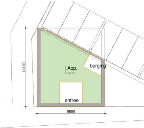
Begane grond
