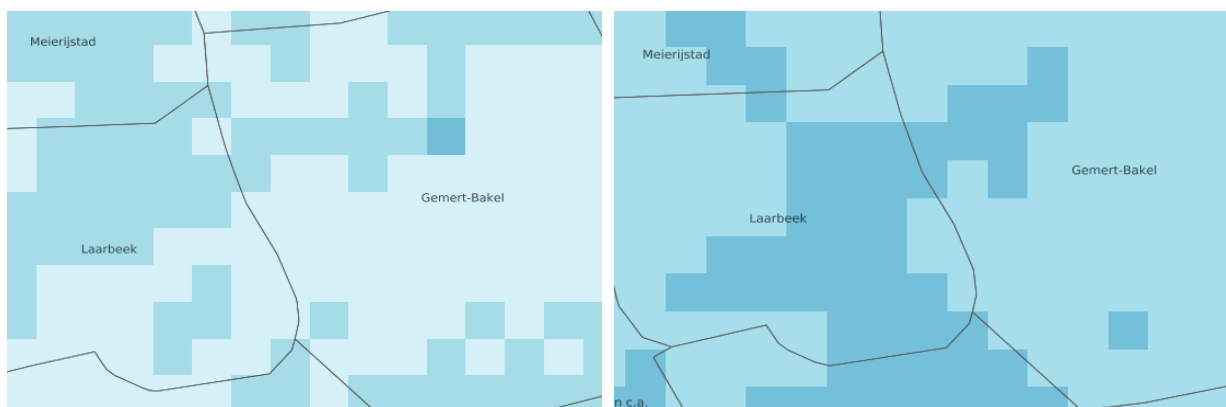
Afbeelding 18. Luchtkwaliteit PM10 (links) en NO2 (rechts) (bron: GCN en GDN 2019)
