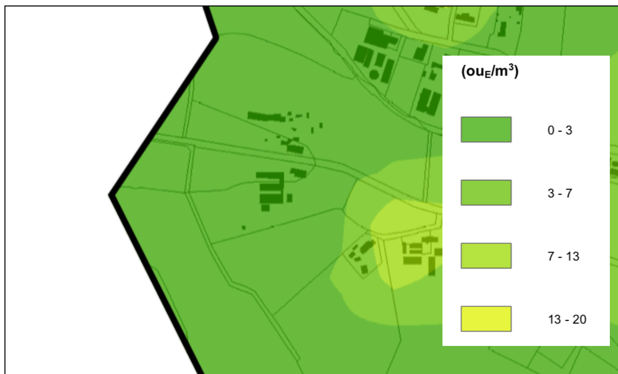
Afbeelding 24. Kaart achtergrondbelasting
