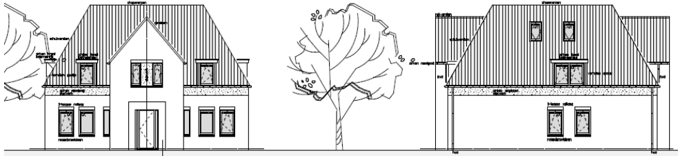
Voorgevel (links) en rechter zijgevel zuidelijke appartementengebouw (Bron: van Santvoort architecten, 2011)
