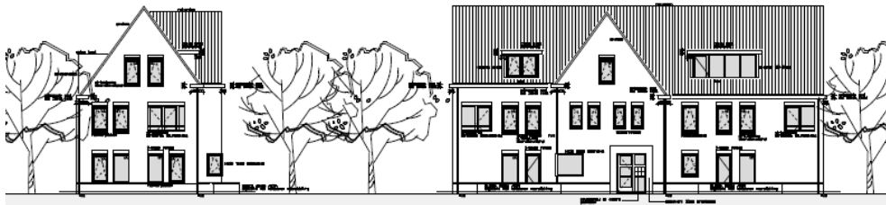
Voorgevel (links) en rechter zijgevel appartementengebouw aan Dorpsstraat (Bron: van Santvoort architecten, 2011)
