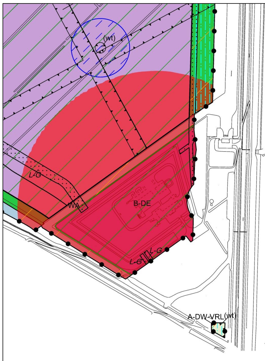
Afbeelding 14. PR 10-6-contour gascompressorstation Spijk
