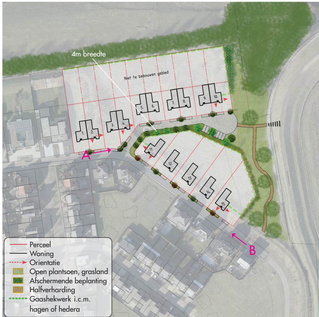
Stedenbouwkundig ontwerp Sleydal Fase 5
