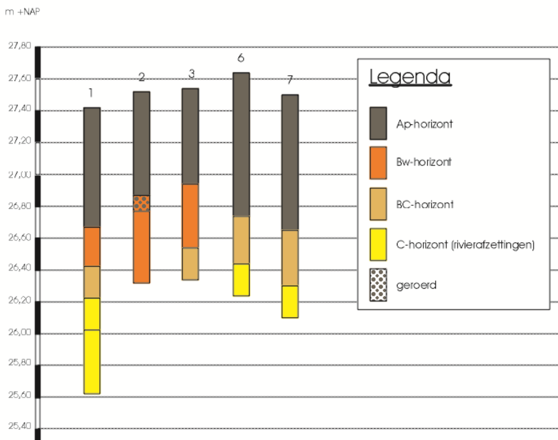
Figuur 18: Boorprofielen
