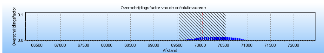
Figuur 4.5 Groepsrisico screening voor A-521 van N.V. Nederlandse Gasunie voor realisatie plan.
