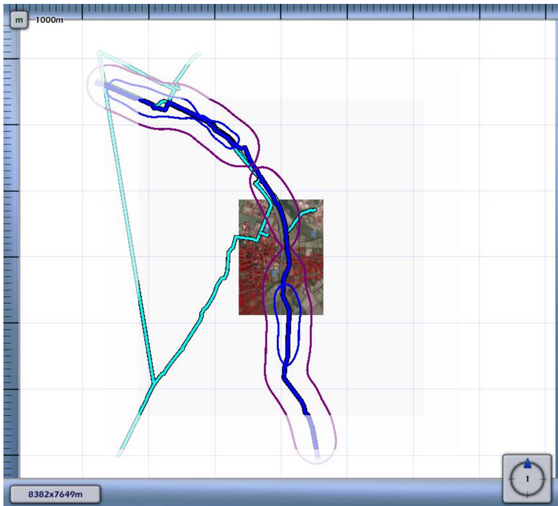
Figuur 3.1 Plaatsgebonden risico voor A-585 van N.V. Nederlandse Gasunie
