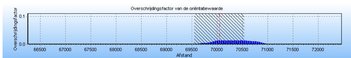
Figuur 4.7 Groepsrisico screening voor A-521 van N.V. Nederlandse Gasunie na realisatie plan.
