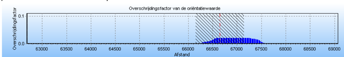
Figuur 4.1 Groepsrisico screening voor A-585 van N.V. Nederlandse Gasunie voor planrealisatie voor realisatie plan.
