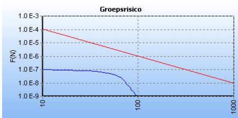
Figuur 5.4 FN curve voor A-521 van N.V. Nederlandse Gasunie voor de kilometer tussen stationing 69550.00 en stationing 70550.00 na realisatie plan.
