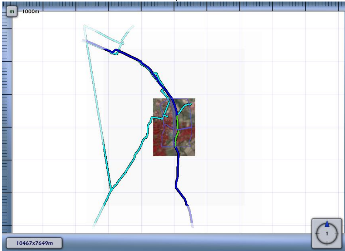
Figuur 4.6 Kilometer leiding behorende bij de maximale overschrijding van de FN-curve voor A-521 van N.V. Nederlandse Gasunie voor realisatie plan.
