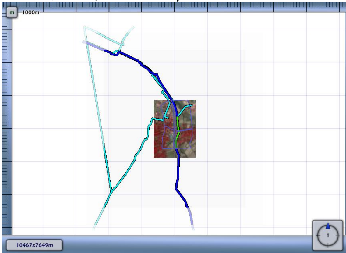
Figuur 4.2 Kilometer leiding behorende bij de maximale overschrijding van de FN-curve voor A-585 van N.V. Nederlandse Gasunie voor realisatie plan.
