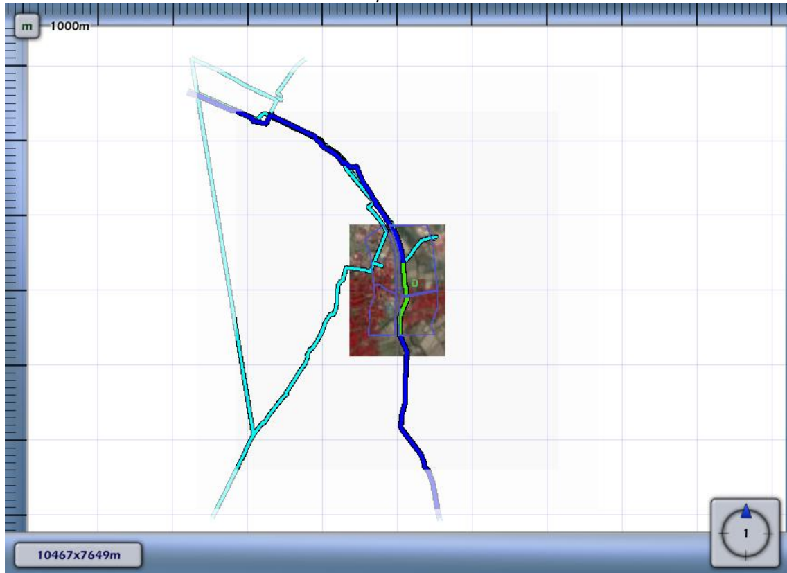
Figuur 4.4 Kilometer leiding behorende bij de maximale overschrijding van de FN-curve voor A-585 van N.V. Nederlandse Gasunie na realistische plan.
