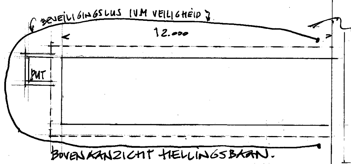
PRINCIPES 1:100
