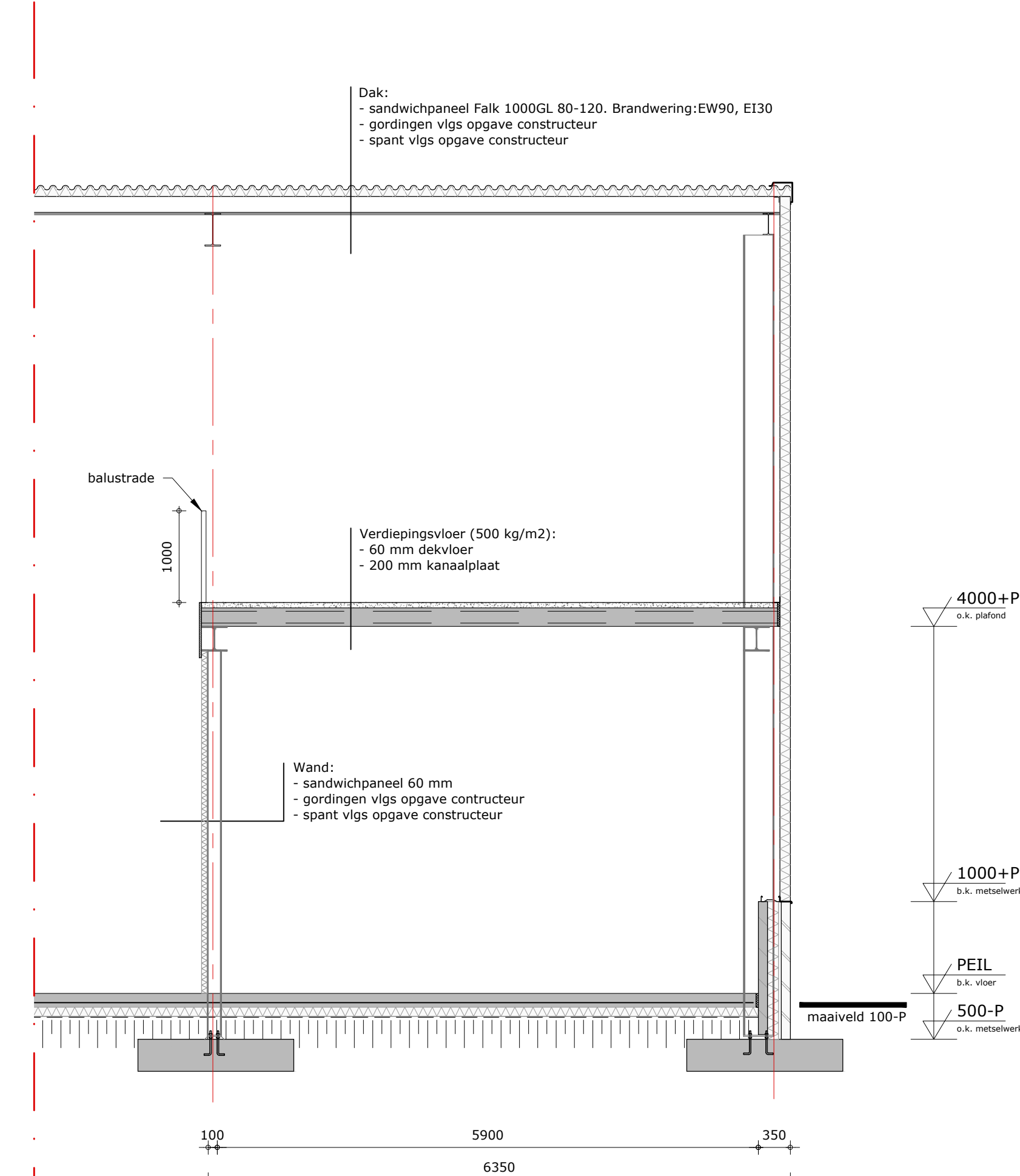
Doorsnede B-B (schaal 1:50)
