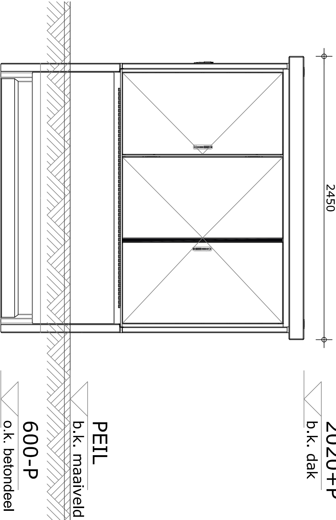
VOORAANZICHT
