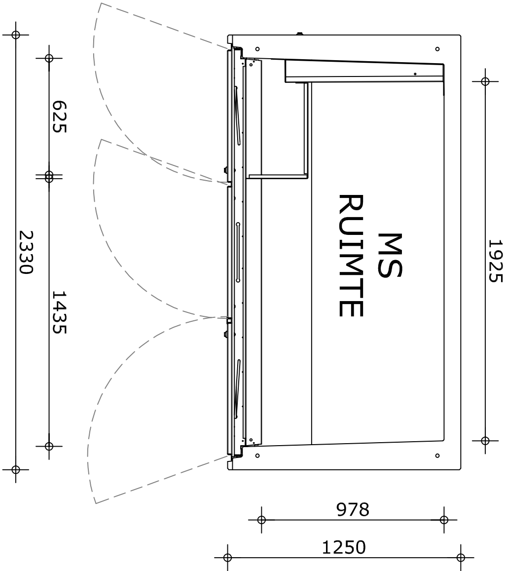
VLOERPLAN
