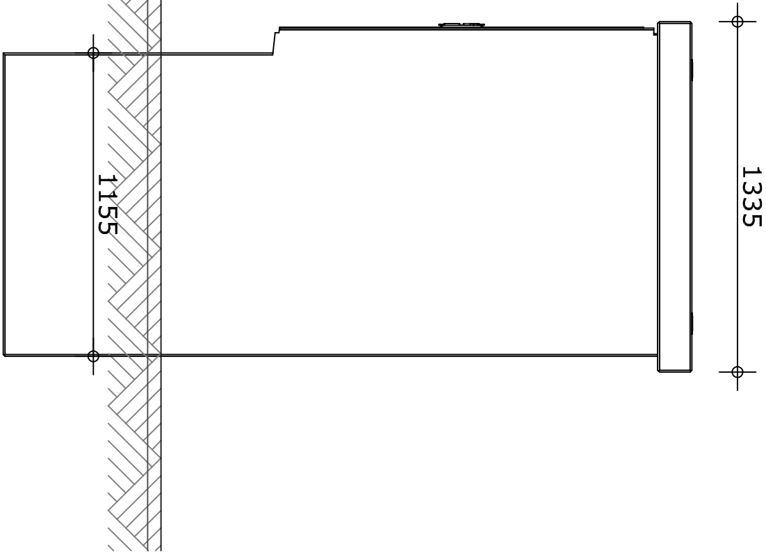
RECHTER ZIJGAANZICHT
