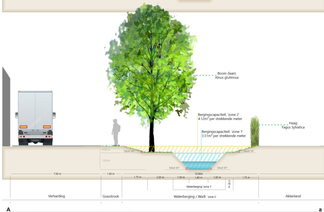
Doorsnede A-a
