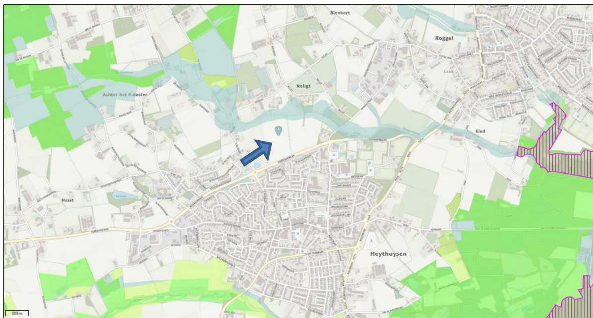
Figuur 10. Ligging goudgroene natuurzone (groen), zilvergroeene natuurzone (geel), bronsgroene natuurzone (blauw) en Natura 2000-gebieden (paars gearceerd) ten opzichte van perceel plangebied (blauwe pijl)
