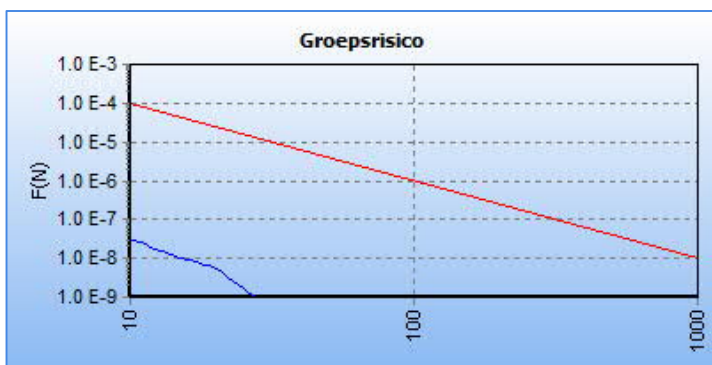
Afbeelding 7 fN-curve buisleiding Z-513-01 deel 1, toekomstige situatie
