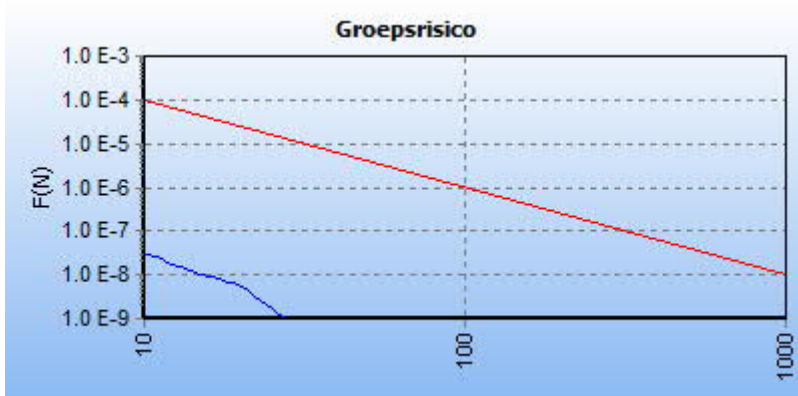
5.2 Figuur 5.2 FN curve voor 7218_leiding-Z-513-01-deel-2 van N.V. Nederlandse Gasunie voor de kilometer tussen stationing 1760.00 en stationing 2760.00
