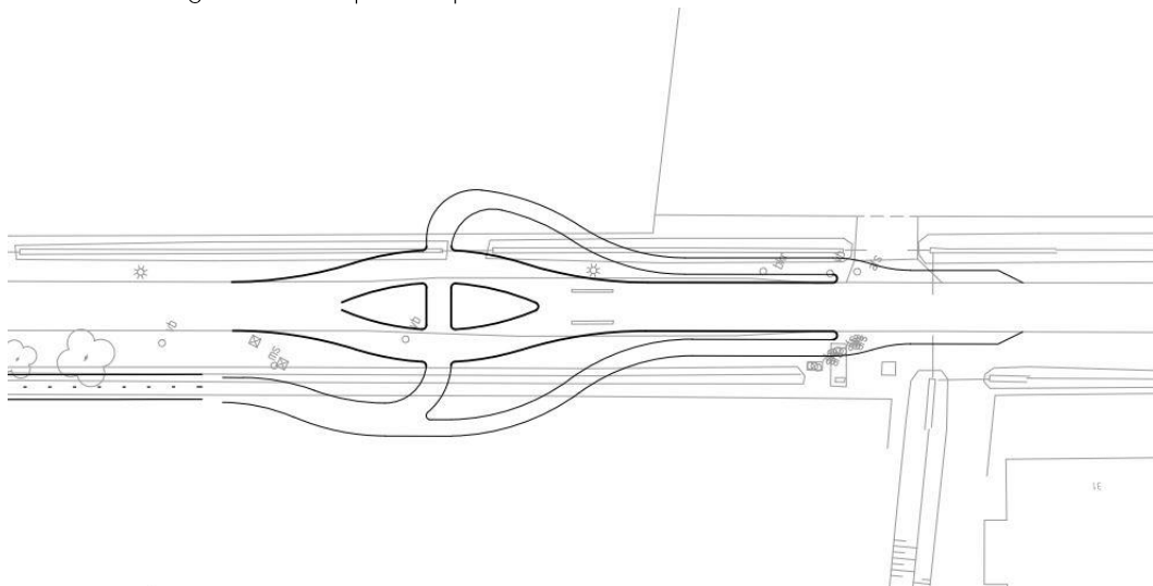
Detail aansluiting en oversteekplaats bij bebouwde kom Neer
