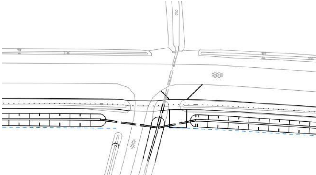
Detail oversteekplaats Heldenseweg op Fort.
