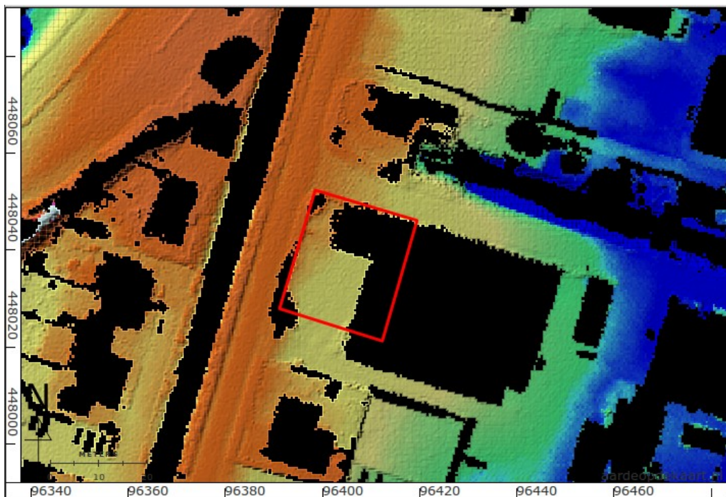
Figuur 9: Plangebied op de hoogtekarte (AHN 2015). Oranje: ca. -1,6 m NAP. Geel : ca. -2m NAP. Blauw: ca. -4,0 m NAP. In zwarte vlakken zijn geen hoogtewaarden beschikbaar (bebouwing, open water).
