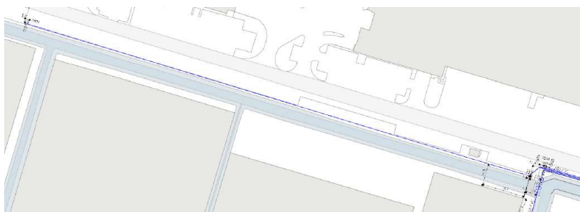
Figuur 18: waterleidingen
