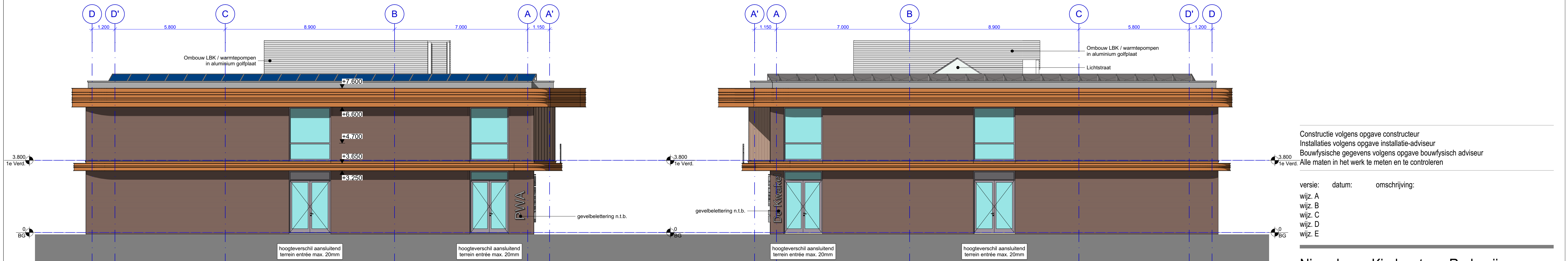
Zuidgevel (Kopgevel PWA)
