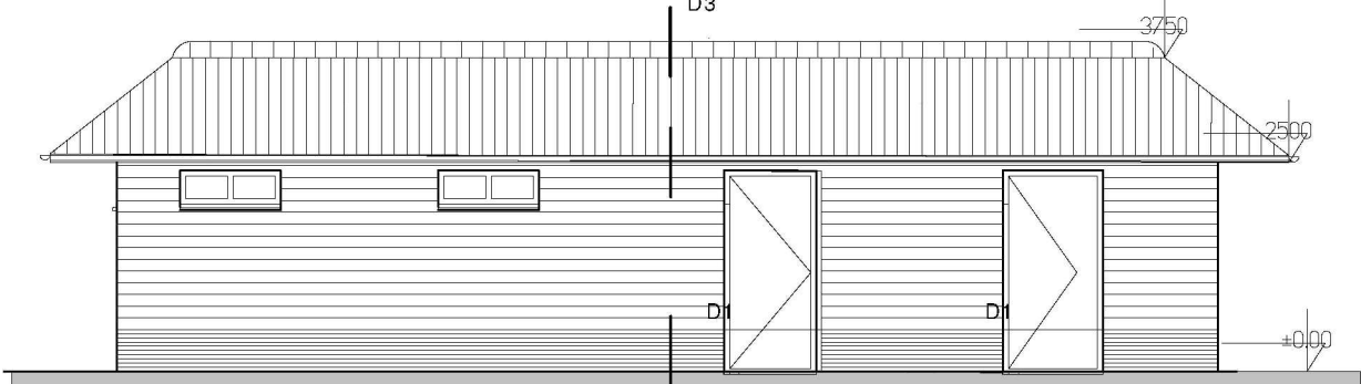
ACHTERGEVEL
