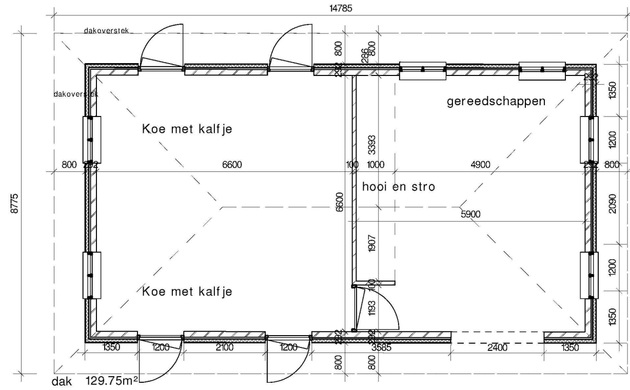
VOORGEVEL KAP
