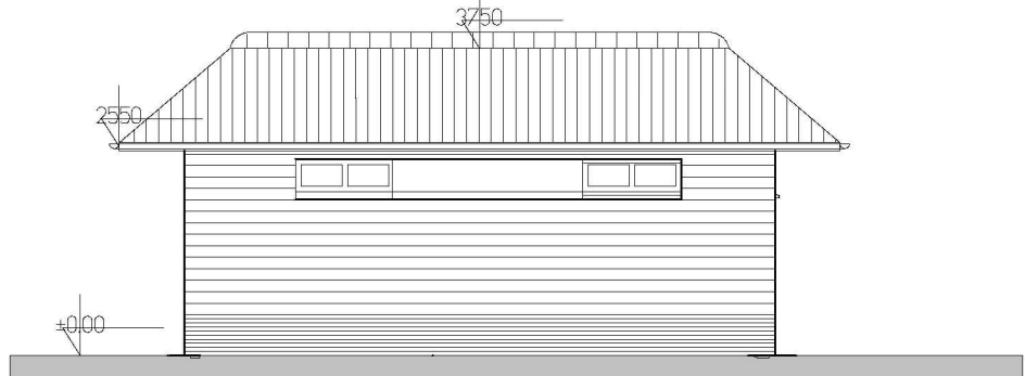
RECHTER ZIJGEVEL
