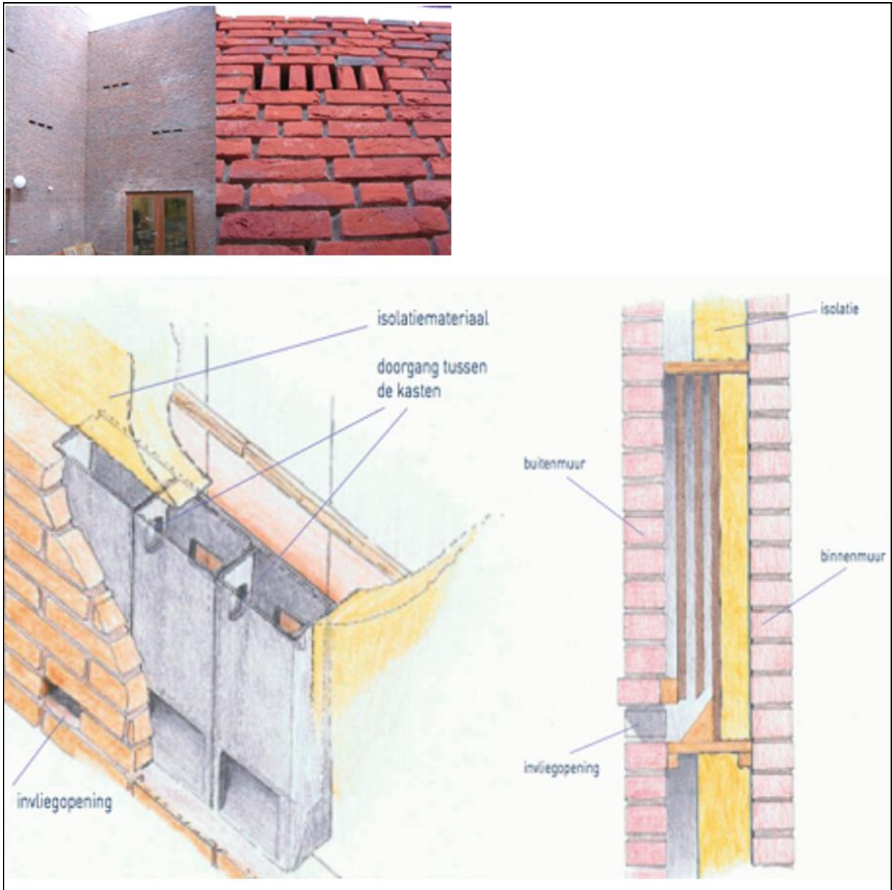
Afbeelding 9: Vrijwel onzichtbare inbouw van vleermuisstenen en technische informatie over de plaatsing daarvan
