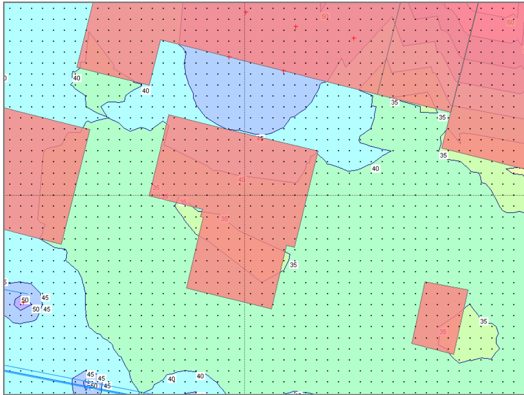
Figuur 4. Geluidcontouren op 1,5 m hoogte voor dagperiode (dBA)
