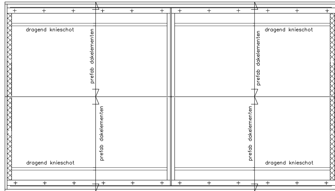
KAPPLAN prefab dakelementen e.e.a. vlg constructeur en leverancier
