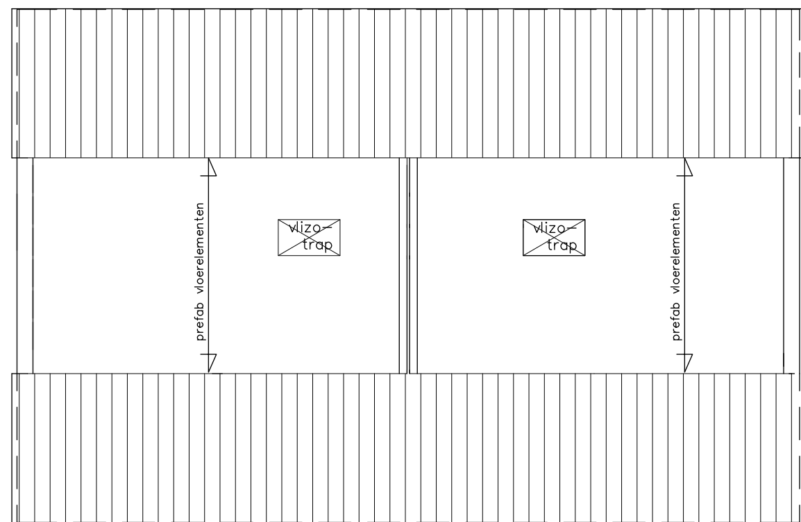
ZOLDERVLOER verdiepingsvloer: prefab vloerelementen e.e.a. vlg constructeur en leverancier
