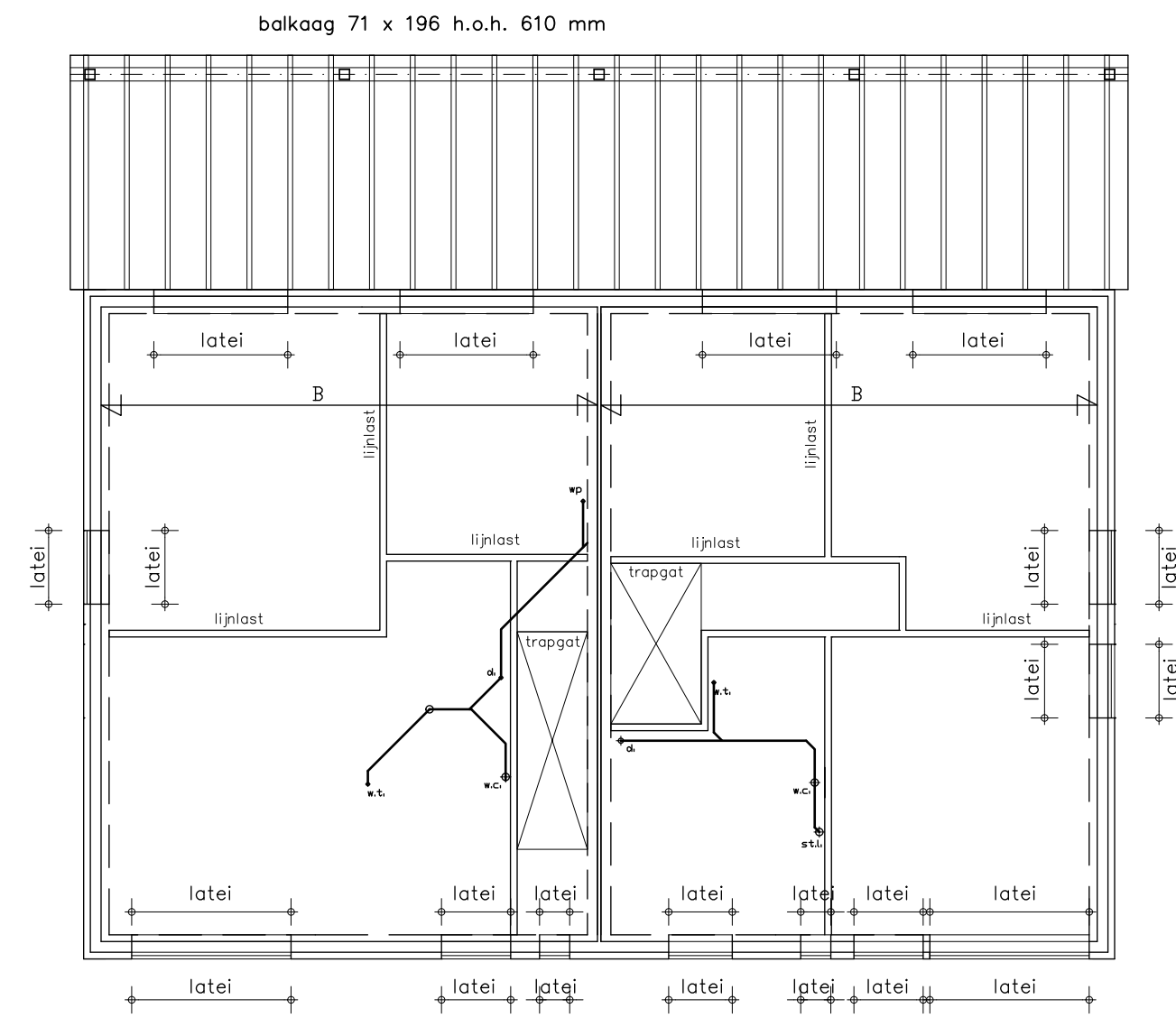
1e verdieping verdiepingsvloer: B= kanaalplaatvloer e.e.a. vlg constructeur lateien: e.e.a. vlg constructeur
