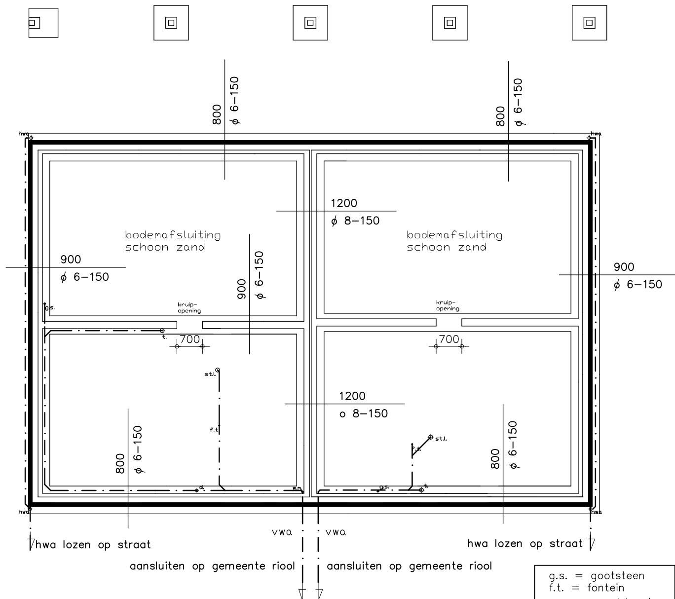
FUNDATIE/RIOLERING fundatie: strokenfundatie e.e.a. vlg berekening en tekening constructeur
