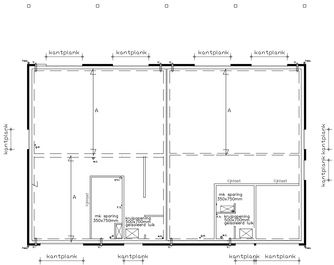
BEGANE GRONDVLOER begane grondvloer: A= geïsoleerde kanaalplaatvloer e.e.a. vlg constructeur Rc: volgens EPN berekening v. = vloerventilatie
