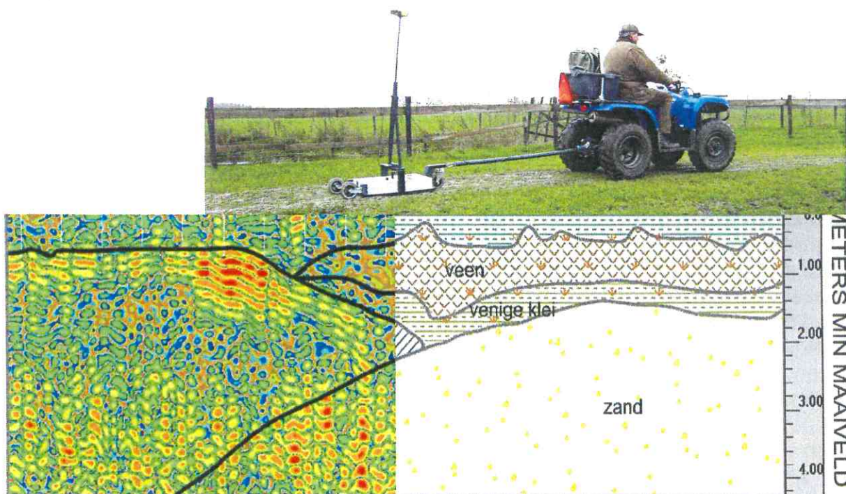
Voorbeeld radarprofiel met bijbehorende interpretatie
