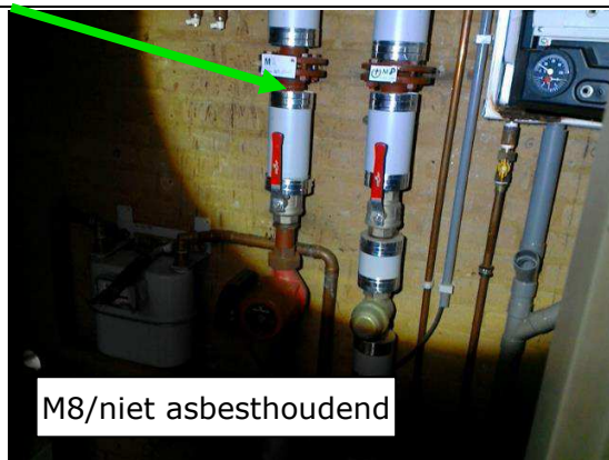
Foto 14 | Flenspakkingen
