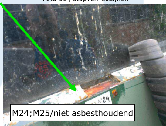
Foto 70 | Stopverf kozijnen
