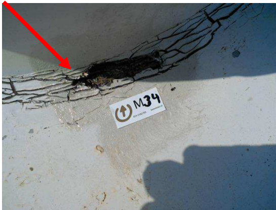
Foto 120 | Kitrand ventilatiekokers op dak
