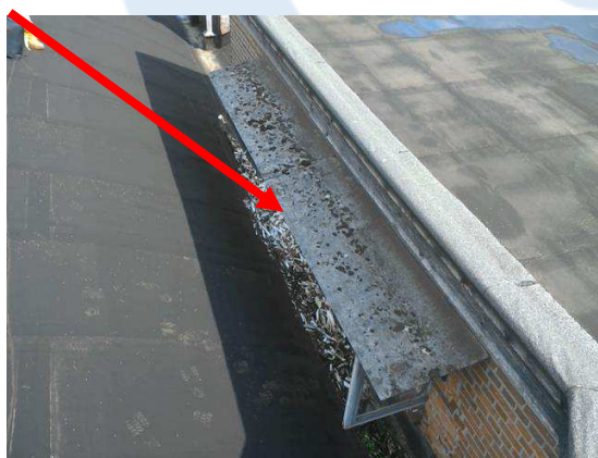
Foto 109 | Beplating zonnescerm
