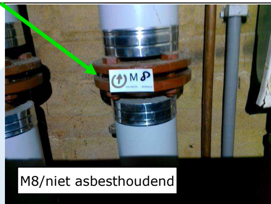
Foto 15 | Flenspakkingen
