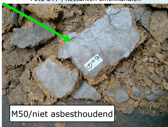
Foto 219 | Restanten Linexkanalen
