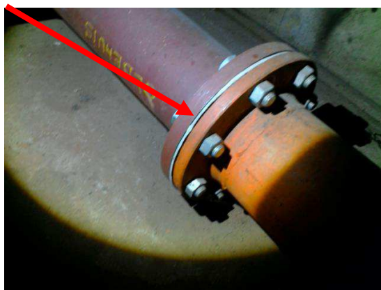
Foto 87 | Flenspakkingen sprinkler installatie
