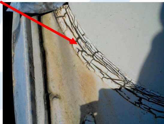
Foto 117 | Kitrand ventilatiekokers op dak
