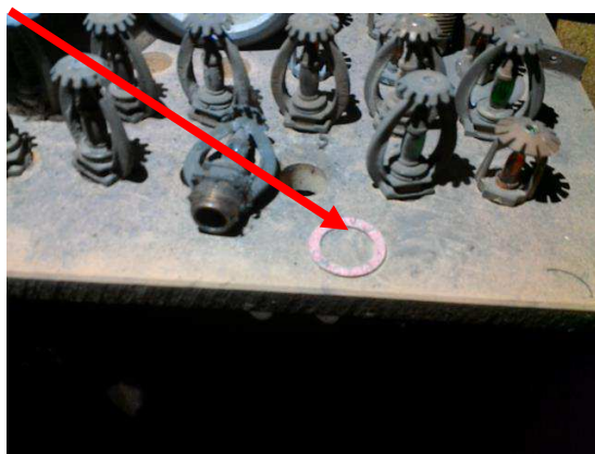
Foto 85 | Restanten flenspakkingen sprinklerruimte
