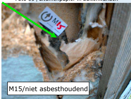
Foto 35 | Bitumenpapier in buitenwanden
