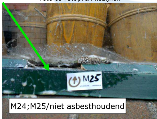
Foto 71 | Stopverf kozijnen
