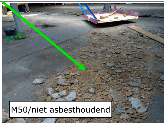
Foto 217 | Restanten Linexkanalen
