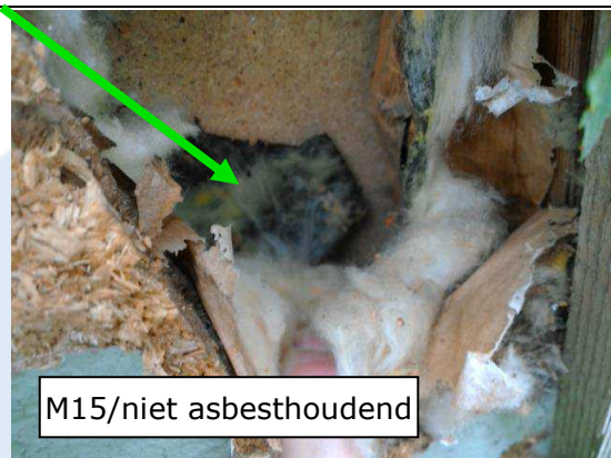
Foto 34 | Bitumenpapier in buitenwanden
