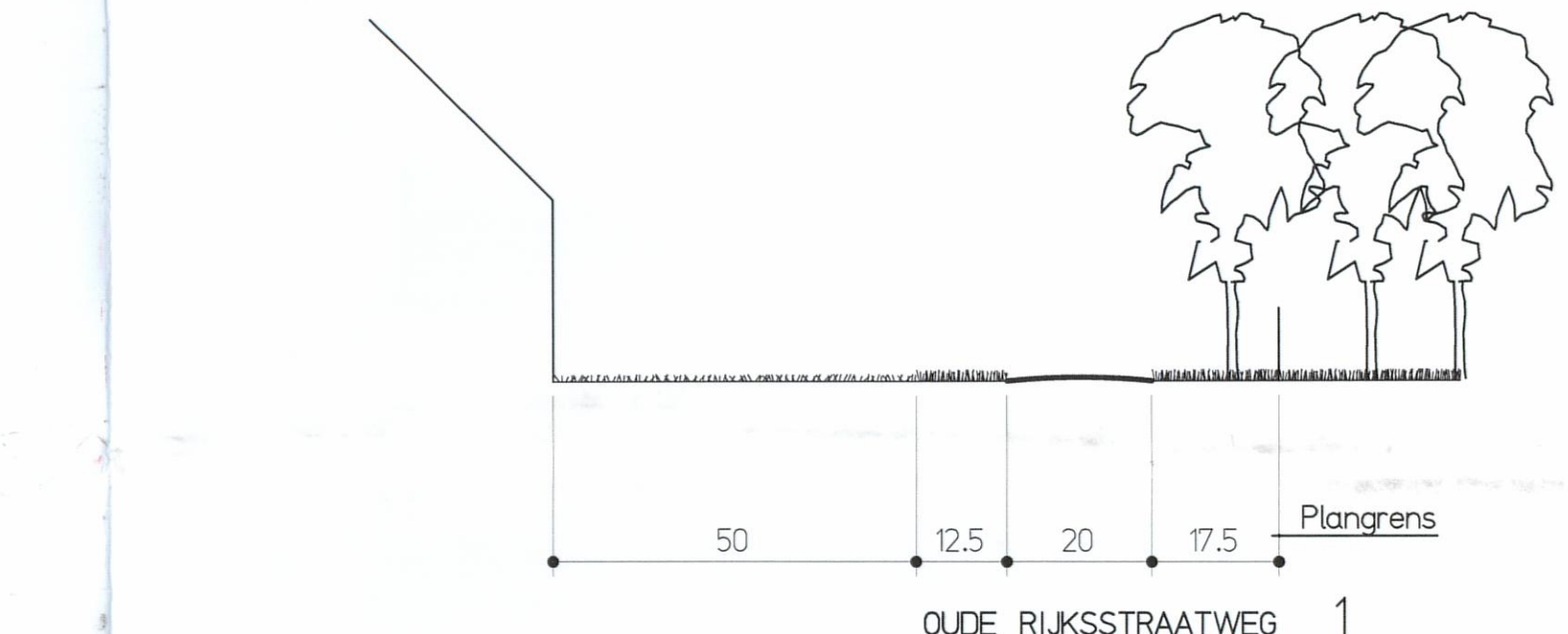
Dwarsprofielen Palmstad/Revius 1:200
