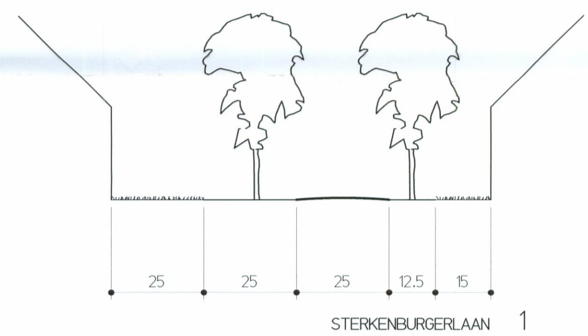
Dwarsprofiel Sterkenburgerlaan 1:200
