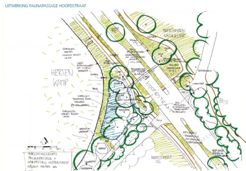
Abbeelding 5 Ligging en inrichting rondom de faunatunnel
