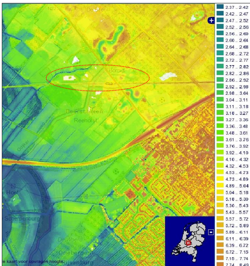
Afbeelding 3: Maaiveldhoogteligging
