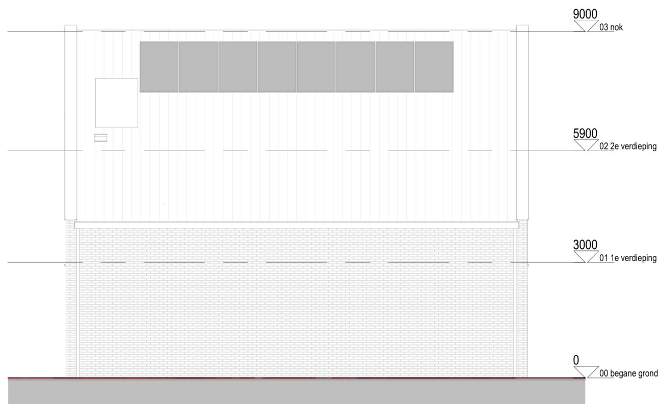
RECHTER ZIJGEVEL
