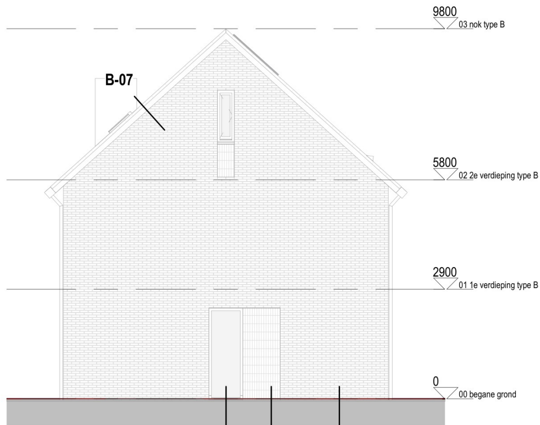
LINKER ZIJGEVEL
