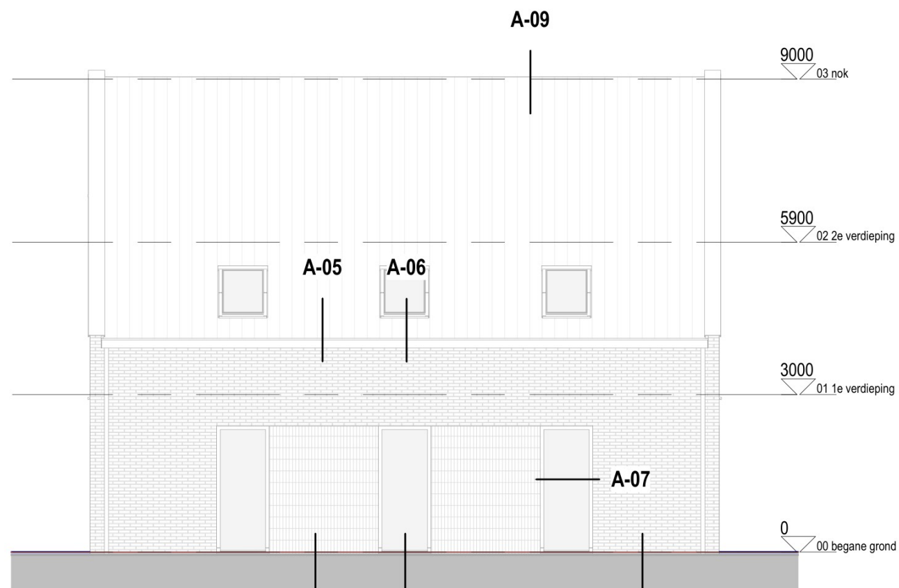
LINKER ZIJGEVEL
