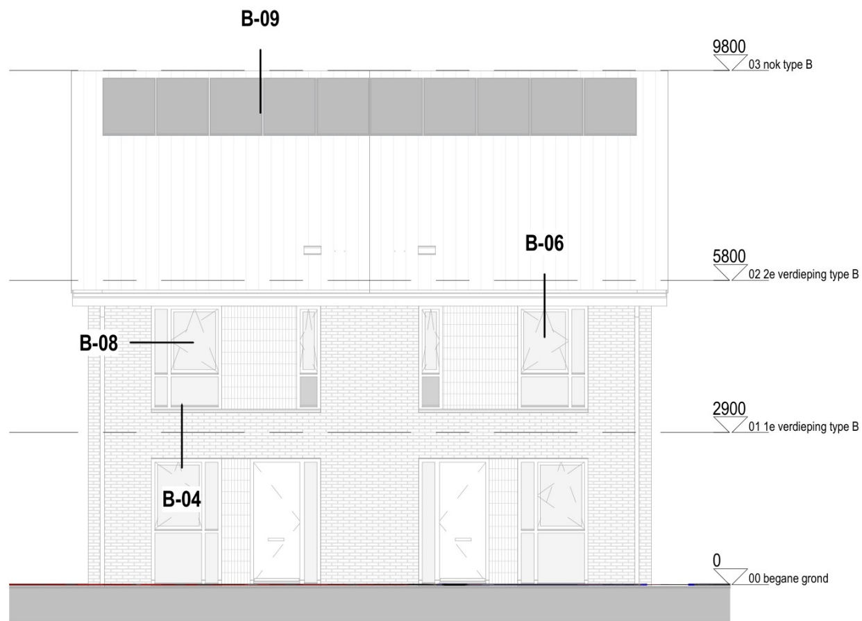
VOORGEVEL
