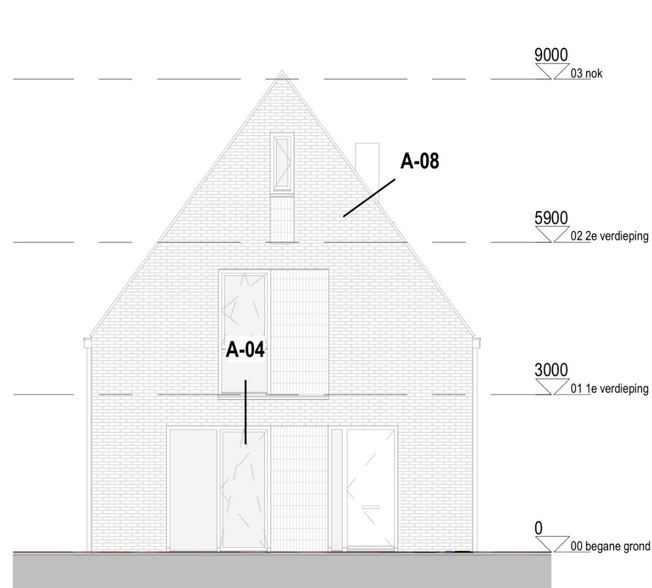
VOORGEVEL
