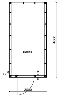
Enkele Berging - Plattegrond
