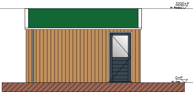
Bergingen - Linkerzijgevel
