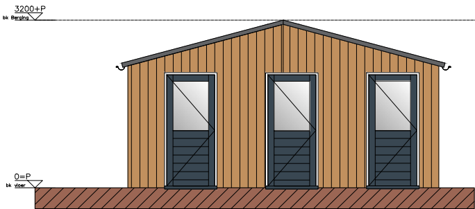
Bergingen - Achtergevel
