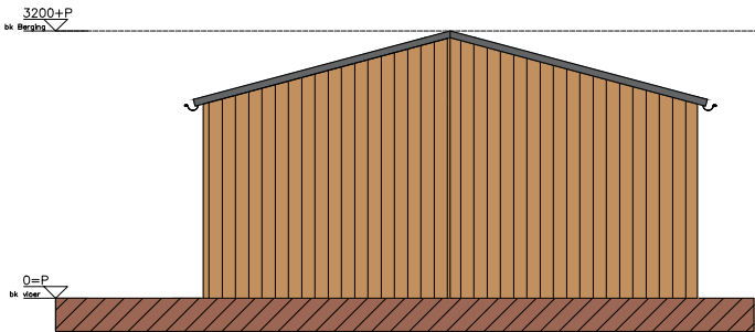
Bergingen - Voorgevel
