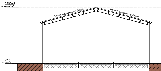
Doorsnede - A-A
