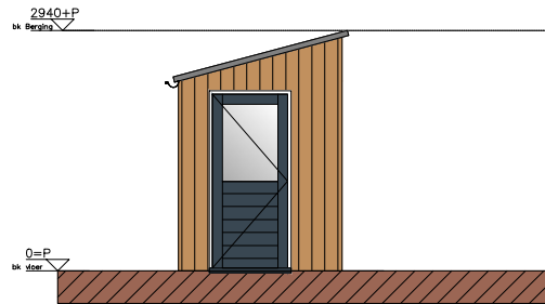
Enkele Berging - Voorzijde
