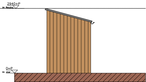
Enkele Berging - Achterzijde
