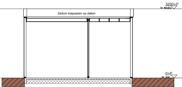
Doorsnede - B-B
