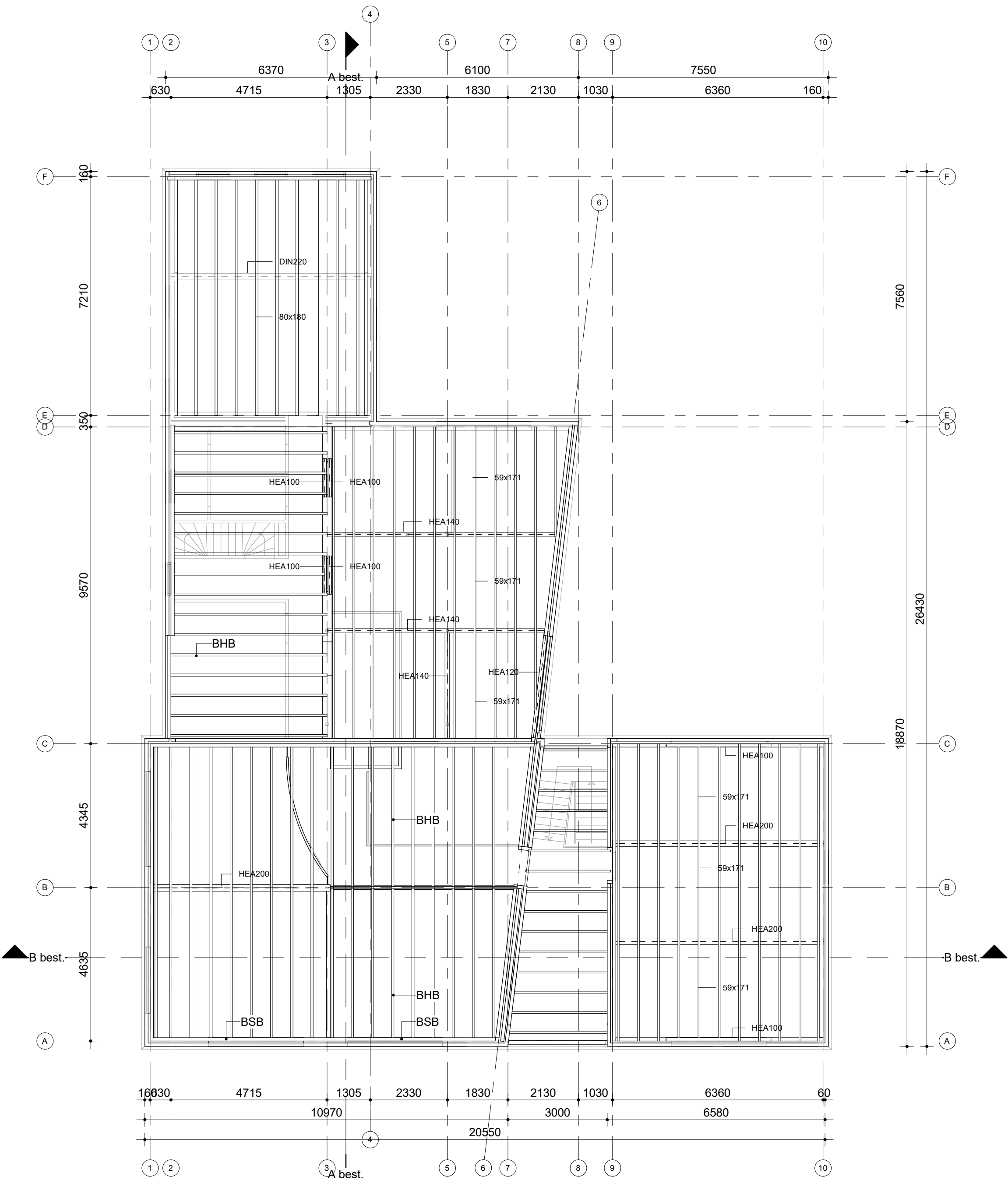
Dakbalklaag bestaande toestand
