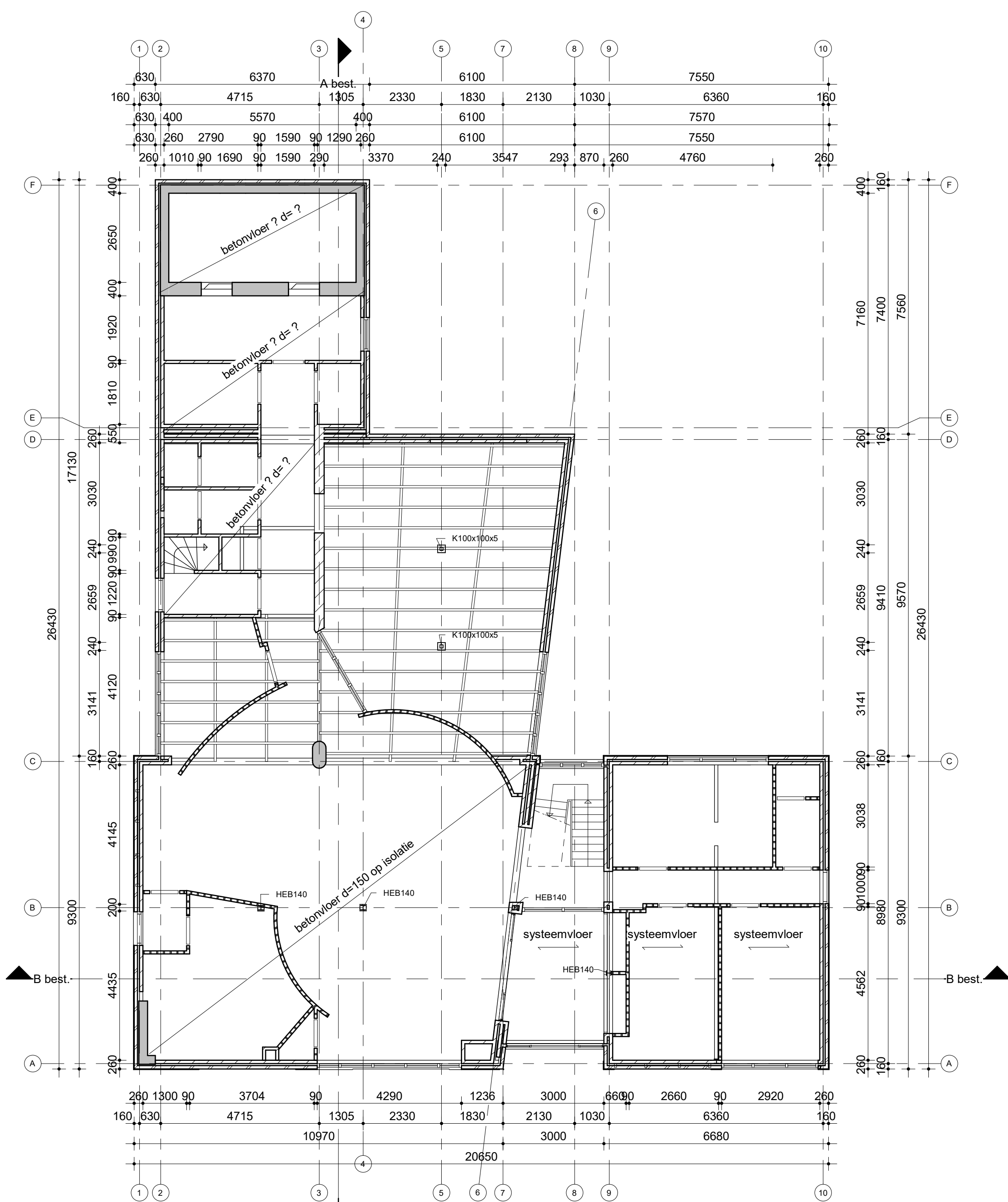
Begane grond bestaande toestand
