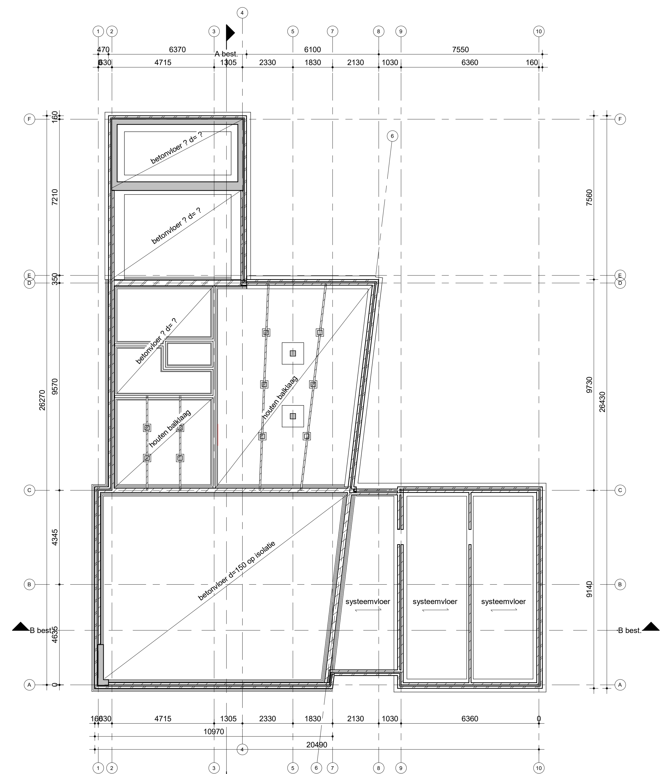
Funderatie bestaande toestand
