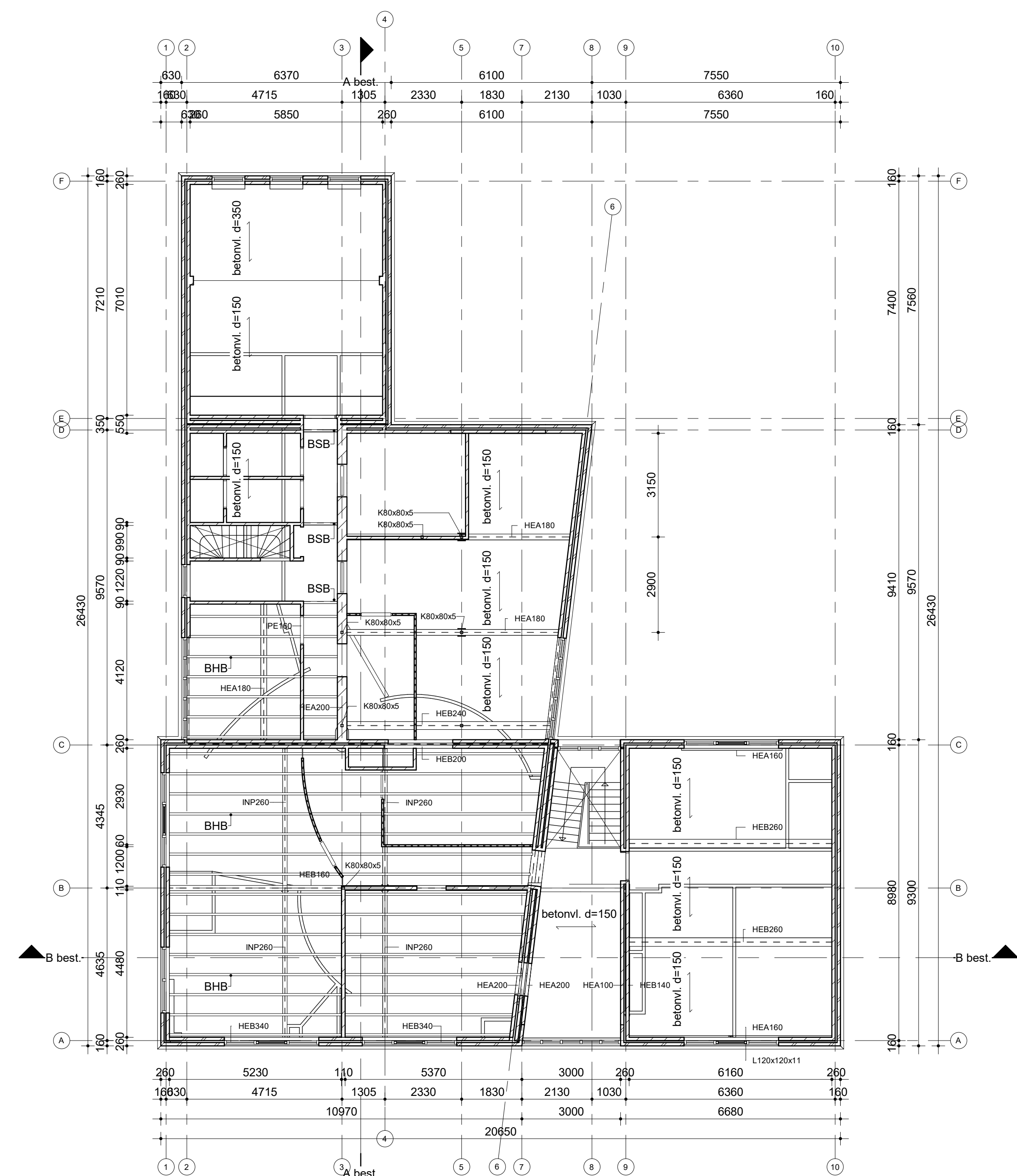
Eerste verdieping balklaag bestaande toestand
