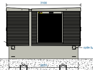
RECHTER ZIJAAANZICHT
