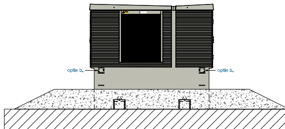
LINKER ZIJAAANZICHT
