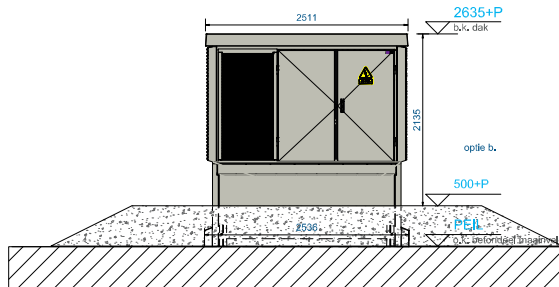
VOORAANZICHT
