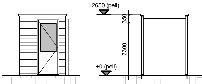
zijgevel doorsnede
