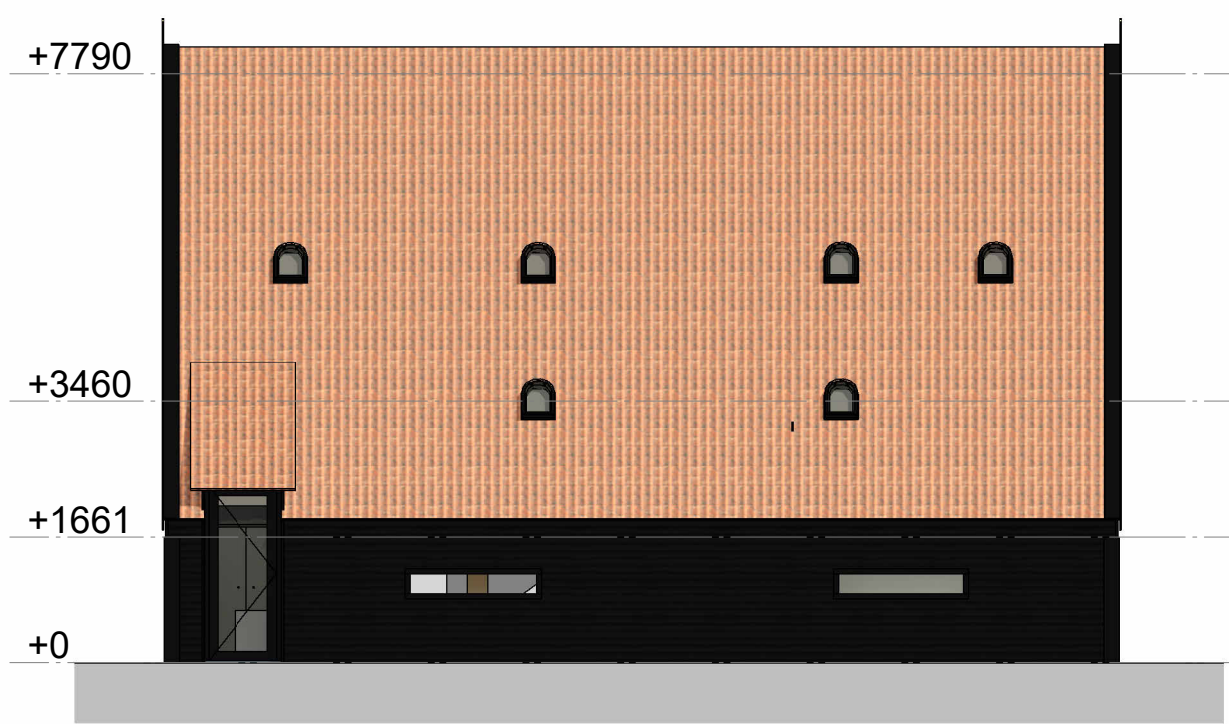
Noordgevel - rechts 1 : 100
