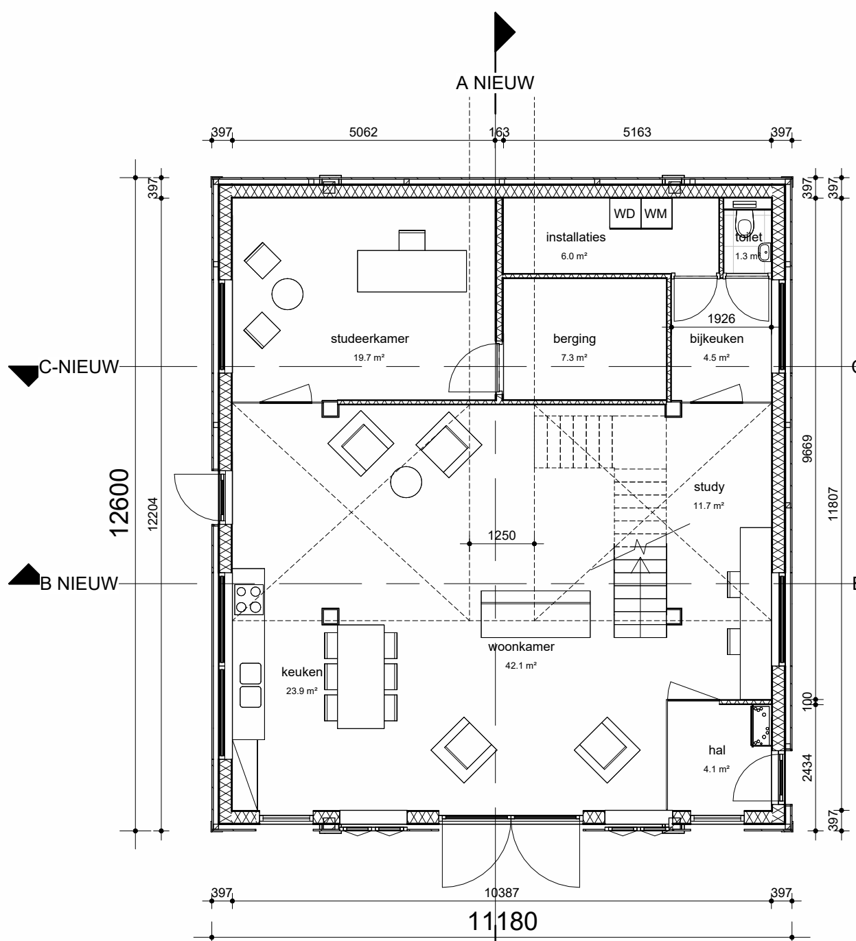
Begane grond 1 : 100
