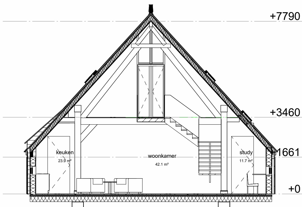
Doorsnede B 1 : 100
