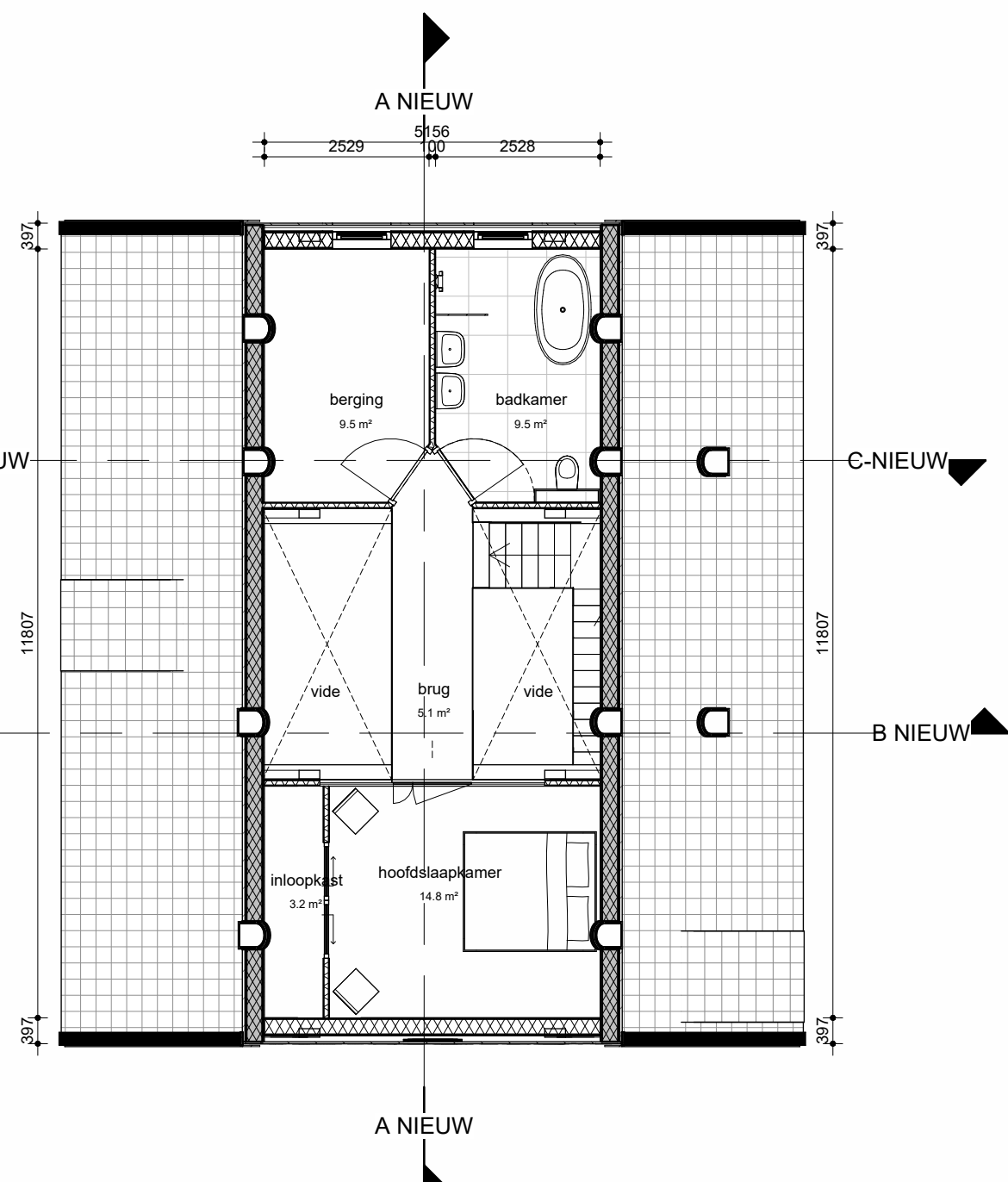
Eerste verdieping 1 : 100
