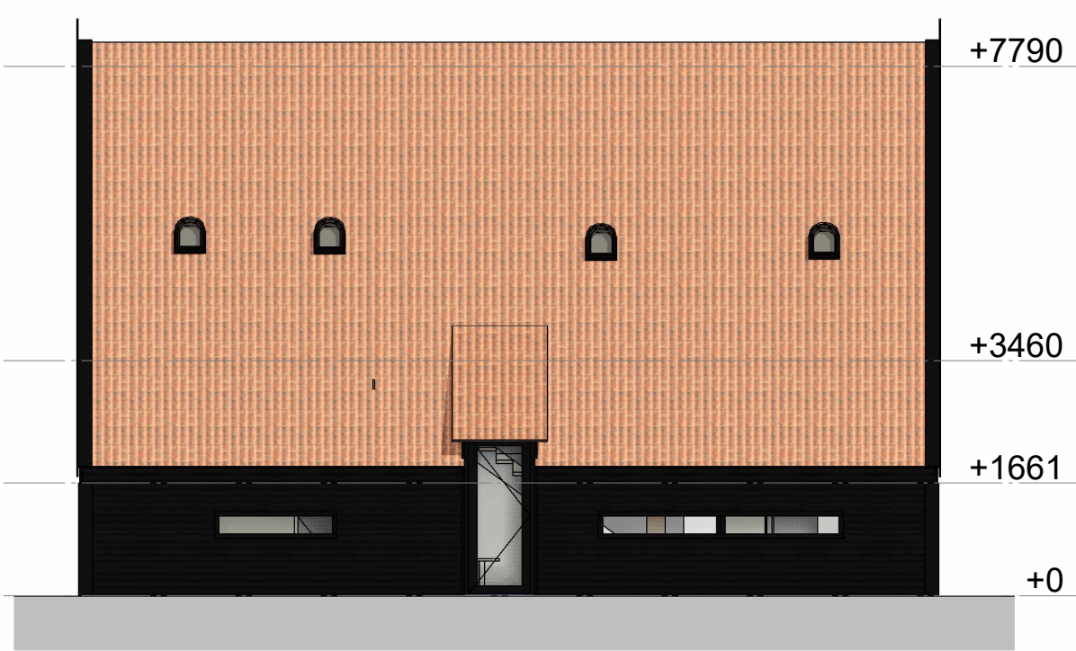
Zuidgevel - links 1 : 100
