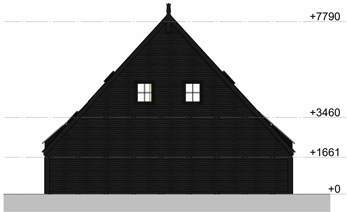
Westgevel - achter 1 : 100
