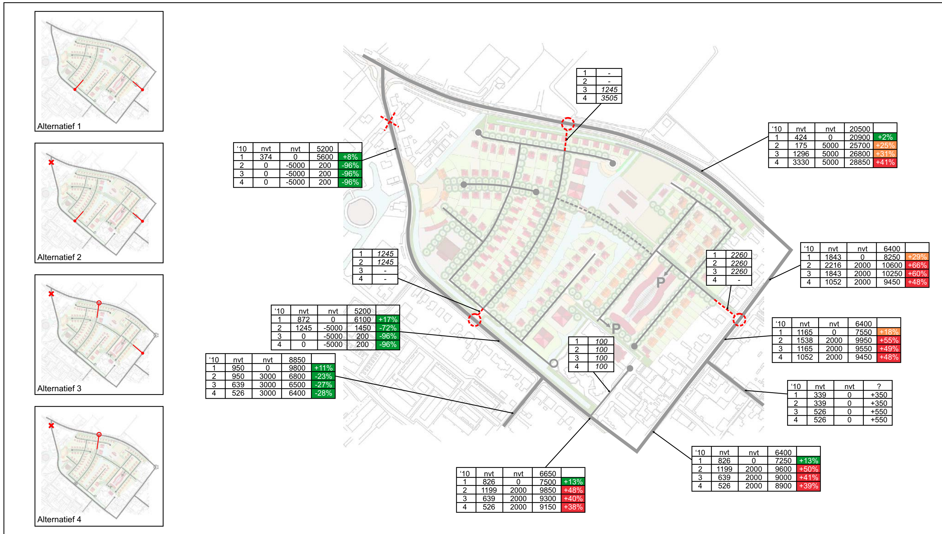
figuur 4 verkeersintensiteiten per alternatief bij gelijke ontsluiting van De Schutse
