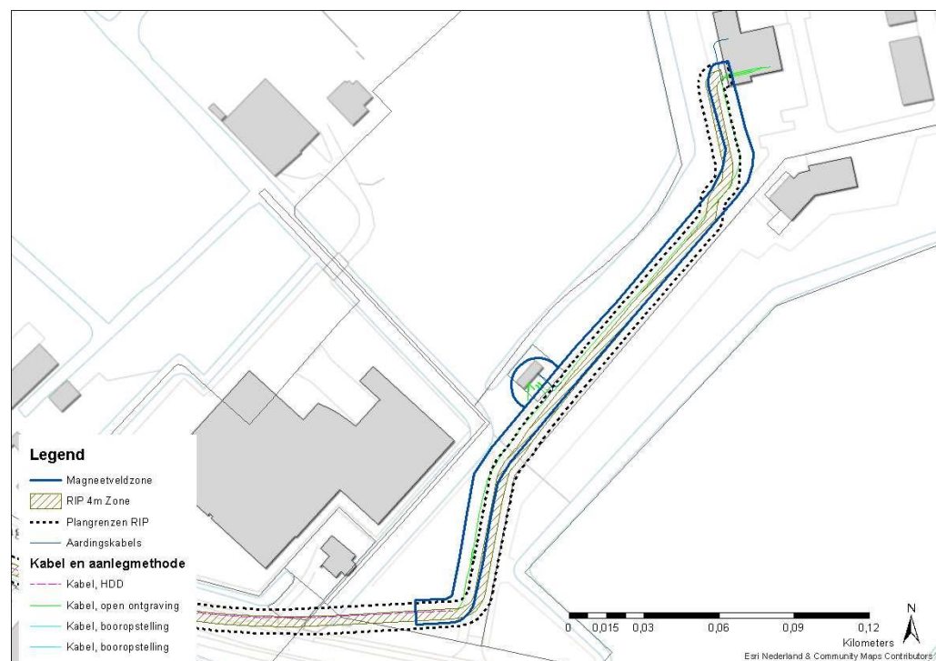
Figuur 4.2 Magneetveldzone afwijking.
