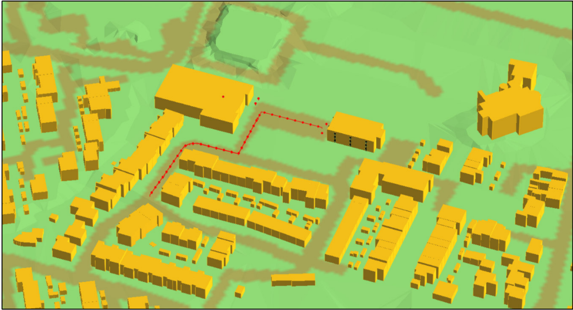
Figuur 3.2: 3D weergave geluidsmodel
