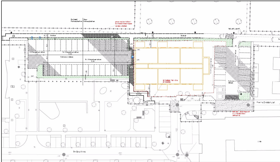
Figuur 3.1: Ontwerp plan 'De Waaier' (concept) met parkeervoorzieningen (Civilink d.d. 04-04-2022)
