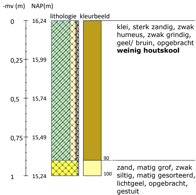
Boring 3 RD-coördinaten: 218779/430120
