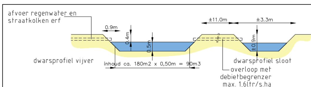
Figuur 14: dwarsprofiel vijver en overloop
