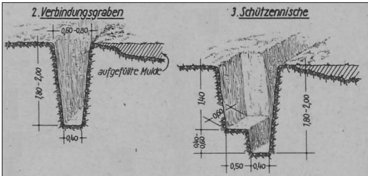
Figuur 19. Doorsnedes van Duitse loopgraven zoals voorgeschreven in de Bildheft für Neuzeitlicher Stellungsbau, 1 juni 1944.
