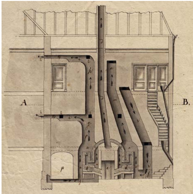
Uitsnede uit de ontwerp-tekening voor het warme luchtverwarmingssysteem, door de architect Übbing (1825)
