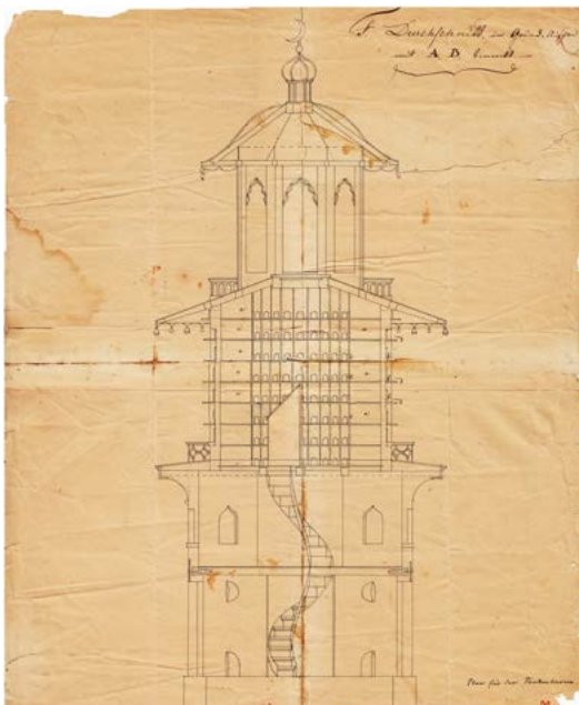
Een van Übbings ontwerpen voor de duiventoren en een foto uit circa 1880 van de gerealiseerde toren
