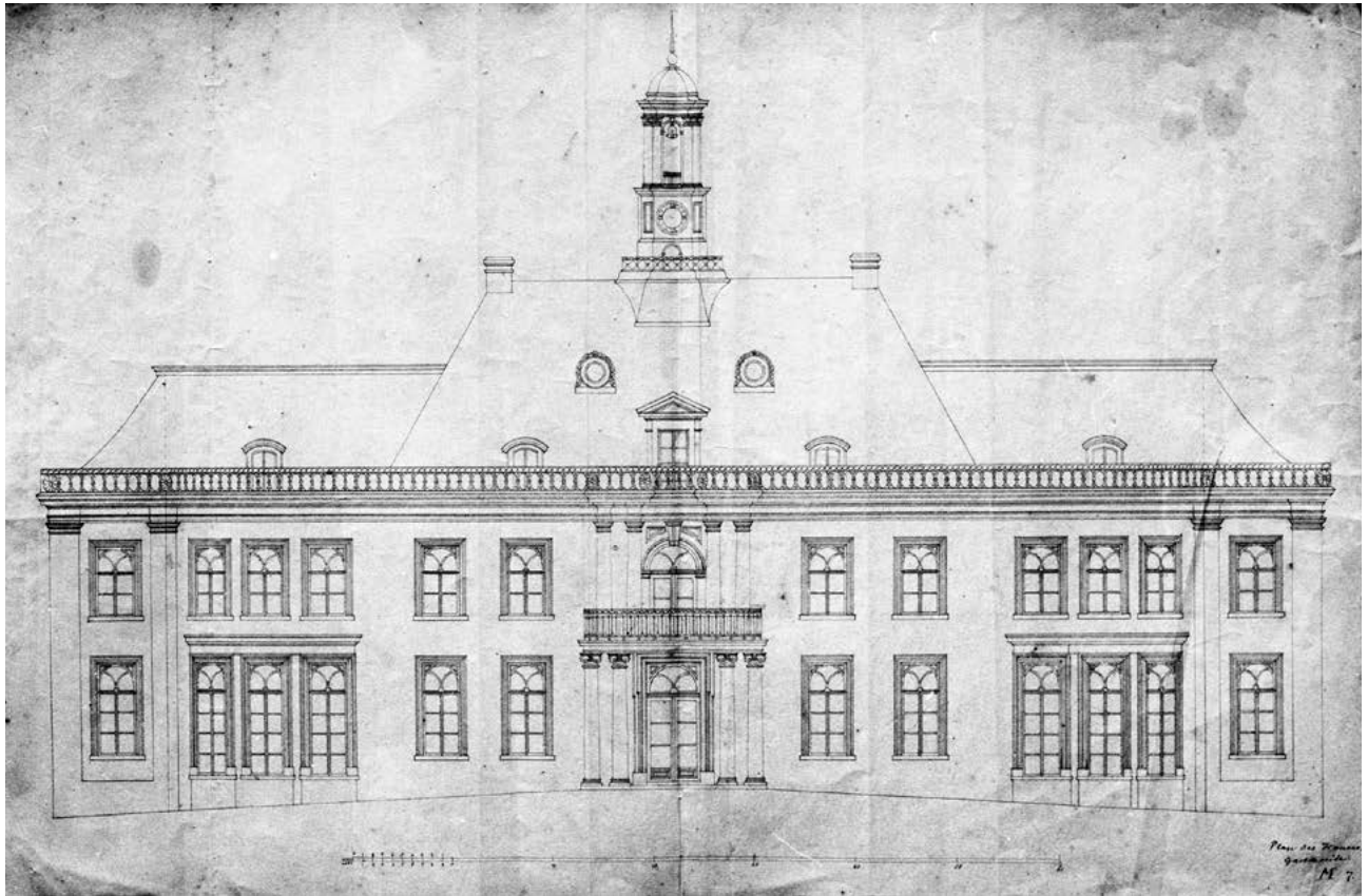
Het ontwerp voor de achtergevel van Landfort, mogelijk door J.D. Zocher jr.
