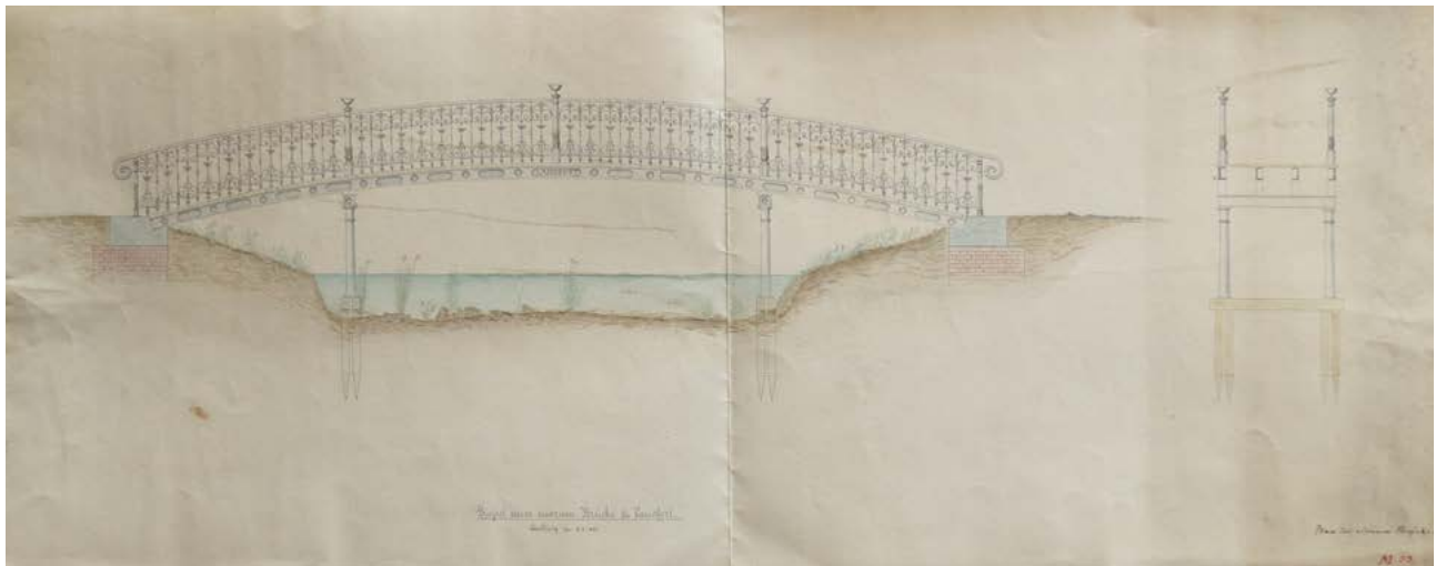
Het ontwerp voor de gietijzeren tuinbrug uit 1872, door ingenieur Carl August Wilhelm Luyken
