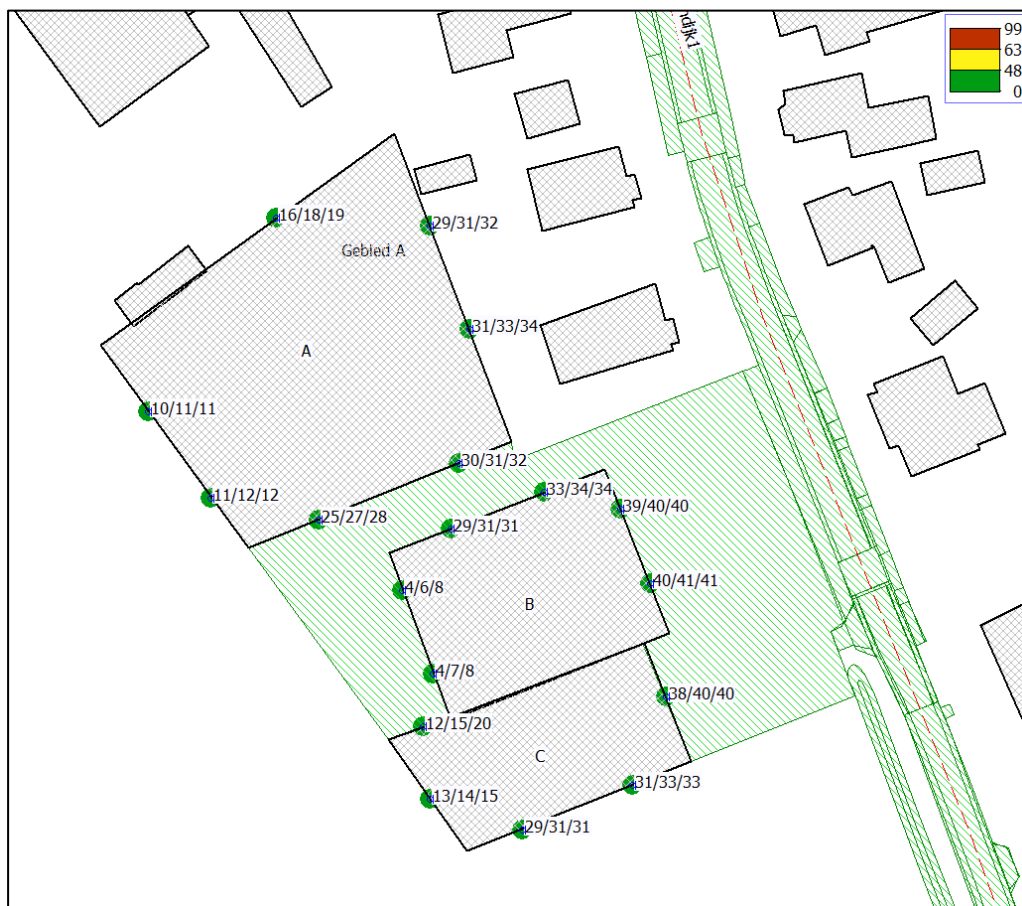
Figuur 7 geluidbelastingen in dB Klompendijk (inclusief aftrek art. 110g Wgh)
