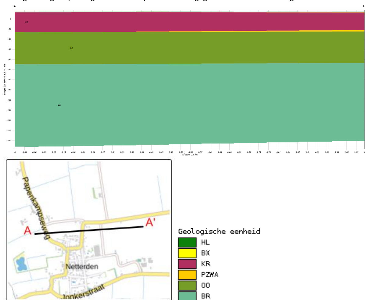
Figuur 1 Geologisch opbouw landelijk model DGM v2.2
