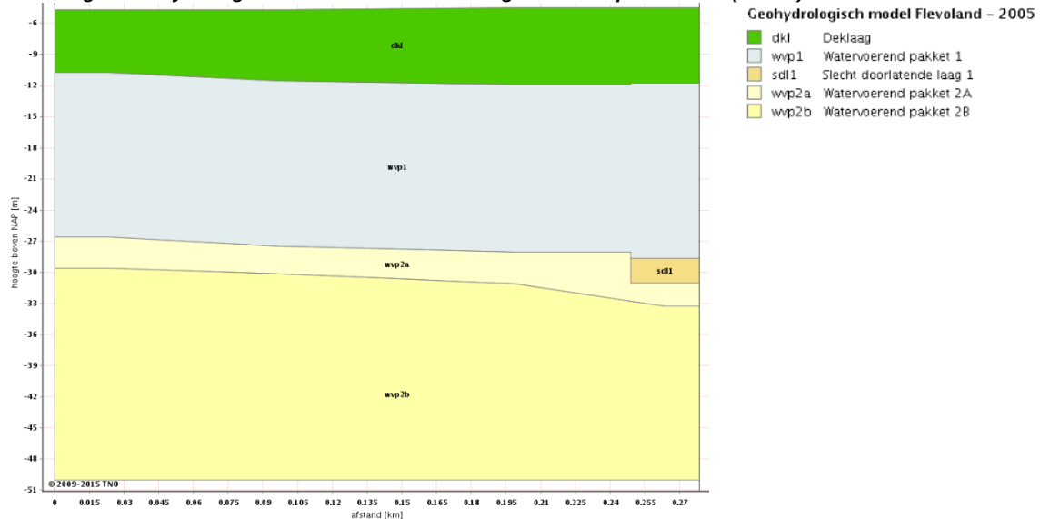
Afbeelding 2: Geohydrologisch model Flevoland -2005 gebaseerd op REGIS II.0 (bron 3)
