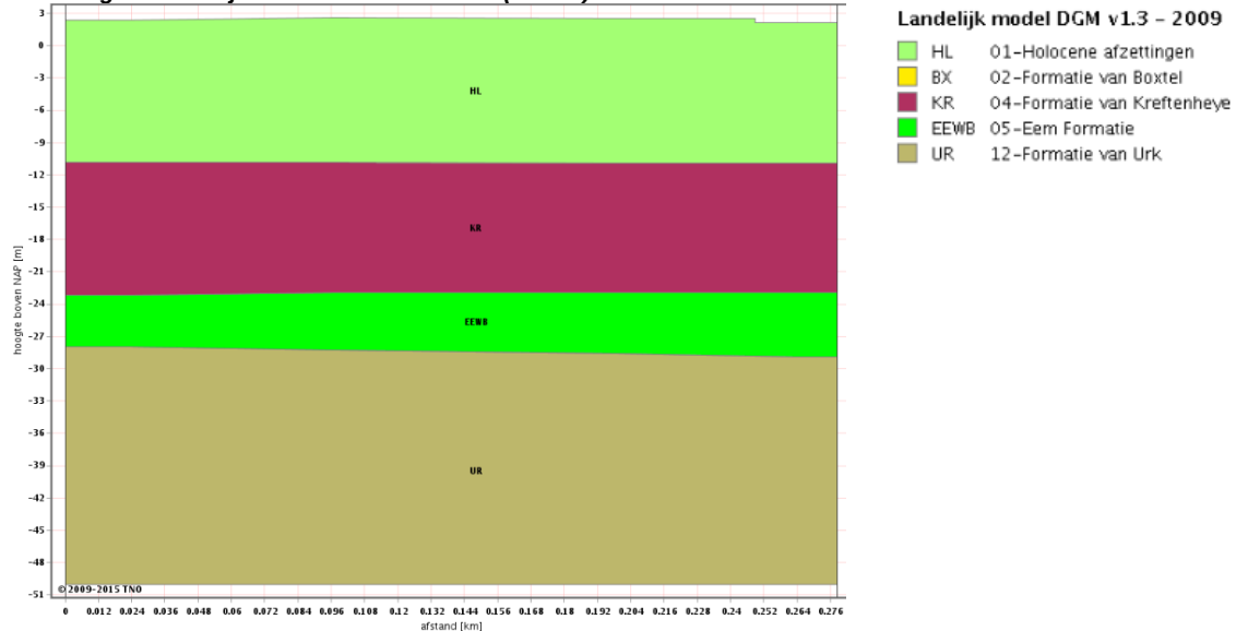
Afbeelding 3: Landelijk model DGM v1.3-2009 (bron 3)
