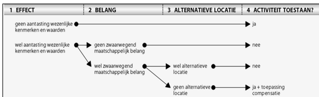
Figuur 4. Schema: Het 'nee, tenzij'-principe van het compensatiebeginsel.
