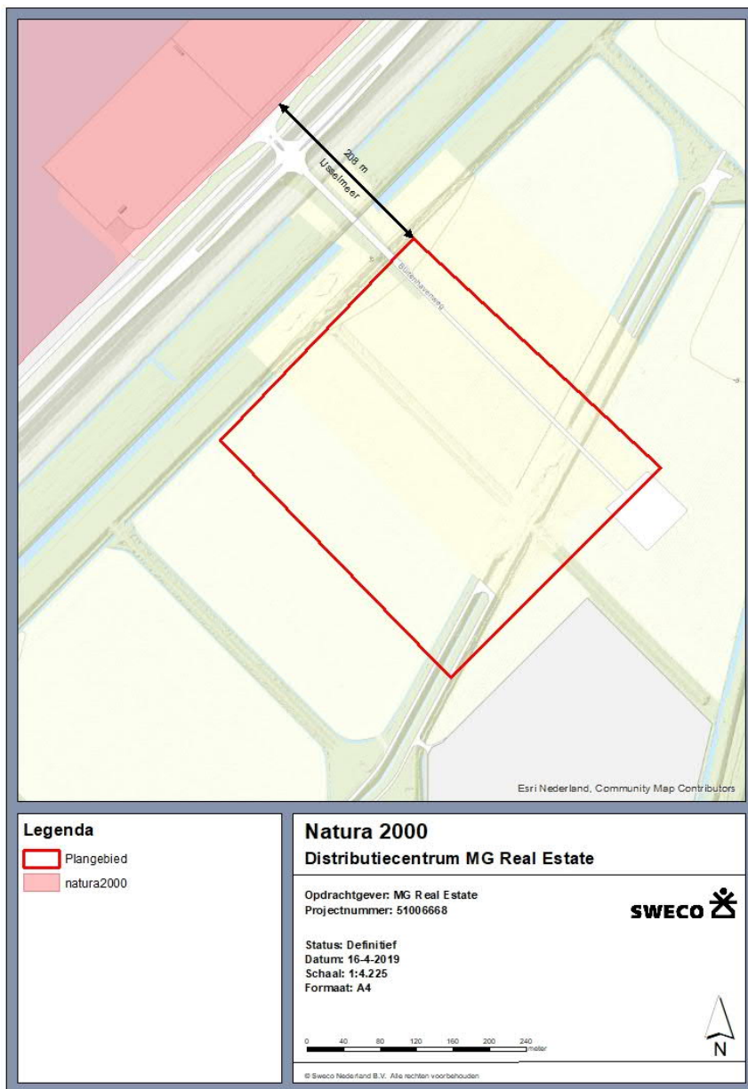
Figuur 2. Ligging plangebied (rode vierkant) t.o.v. het dichtstbijzijnde Natura 2000-gebied.
