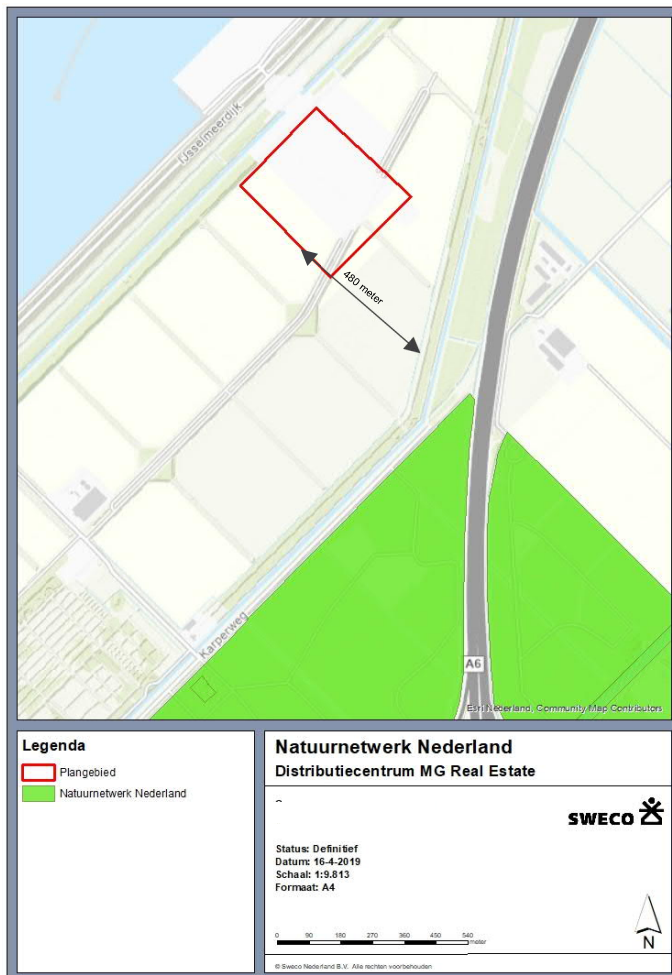
Figuur 5. Ligging plangebied t.o.v. NNN-gebieden (aangegeven in groen).
