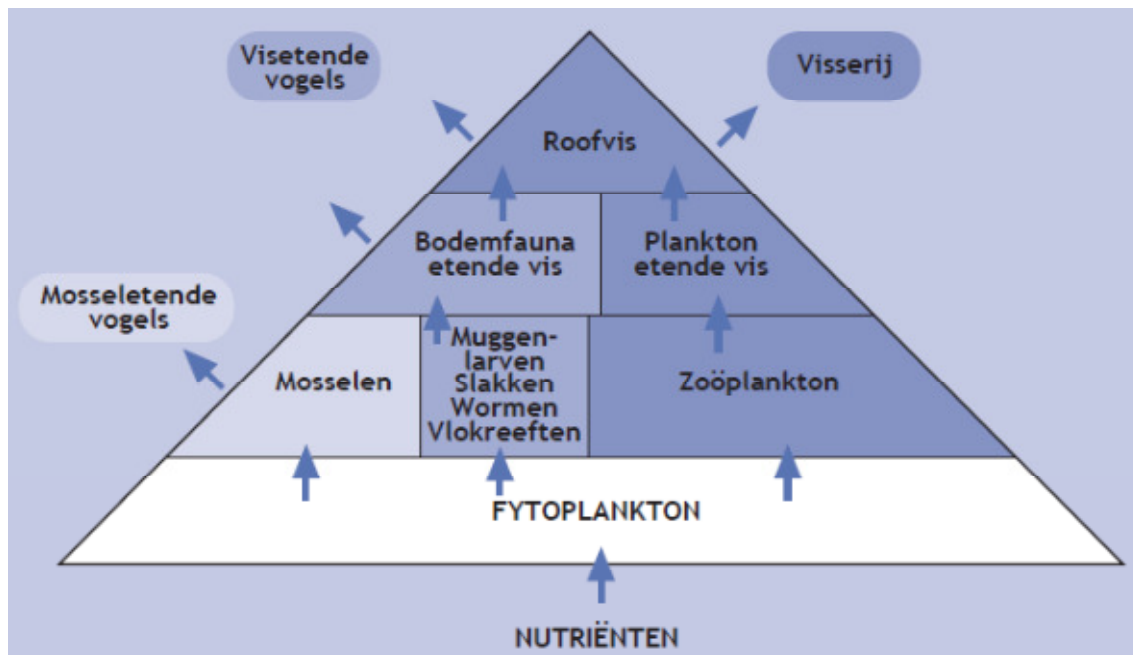
Figuur 5.1 Versimpeld voedselweb van het Markermeer &amp; IJmeer (RIZA, 1998)
